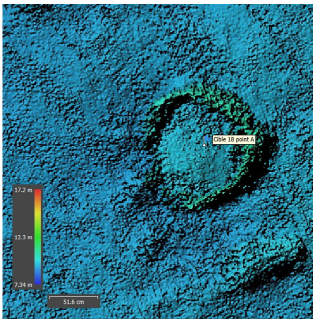
HQ SS MBES Cible 18
