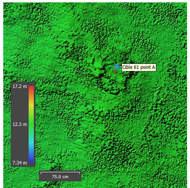
HQ SS MBES Cible 61
