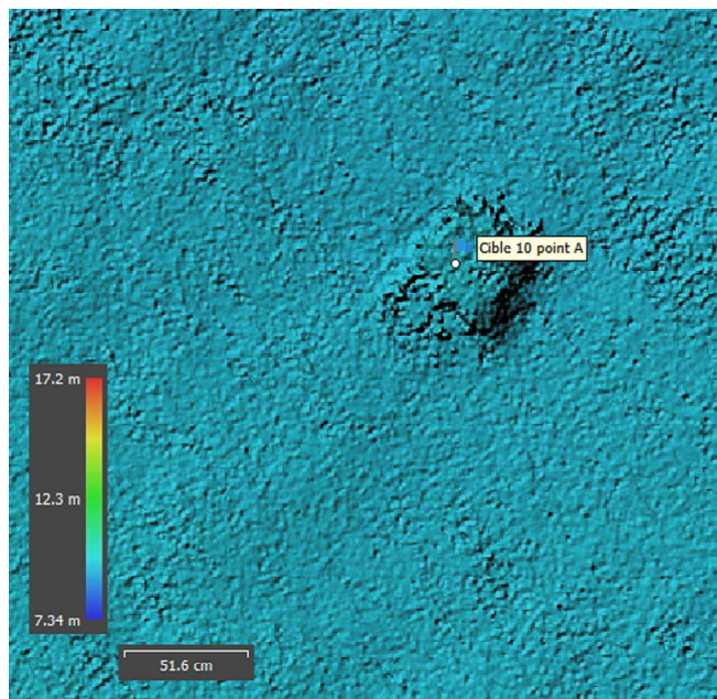
HQ SS MBES Cible 10
