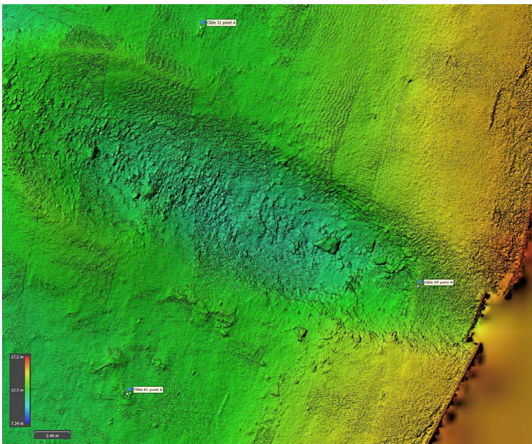
HQ SS MBES Cible 69
