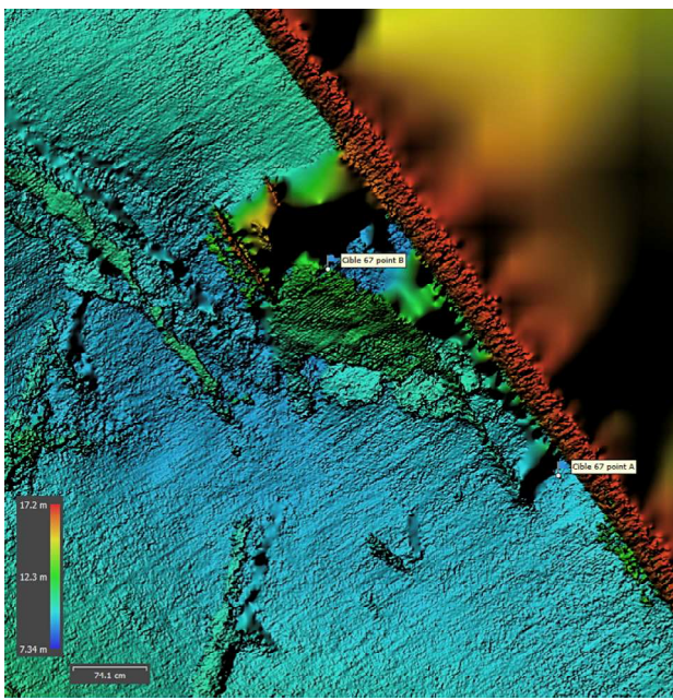
HQ SS MBES Cible 67
