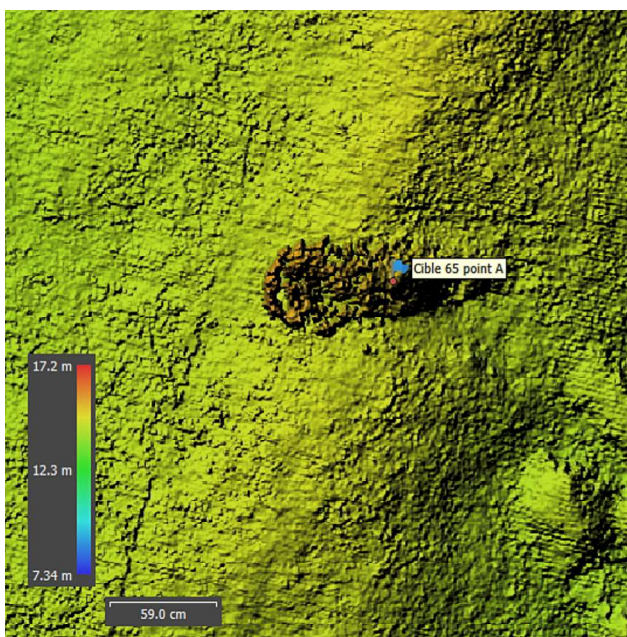
HQ SS MBES Cible 65
