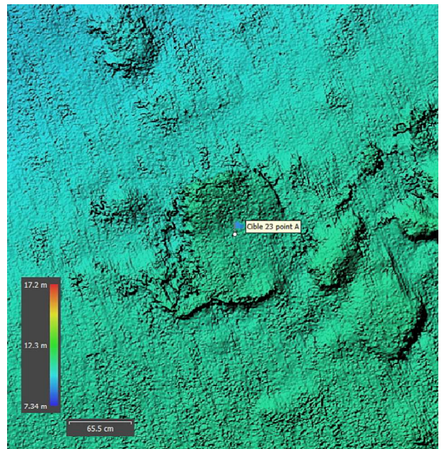
HQ SS MBES Cible 23
