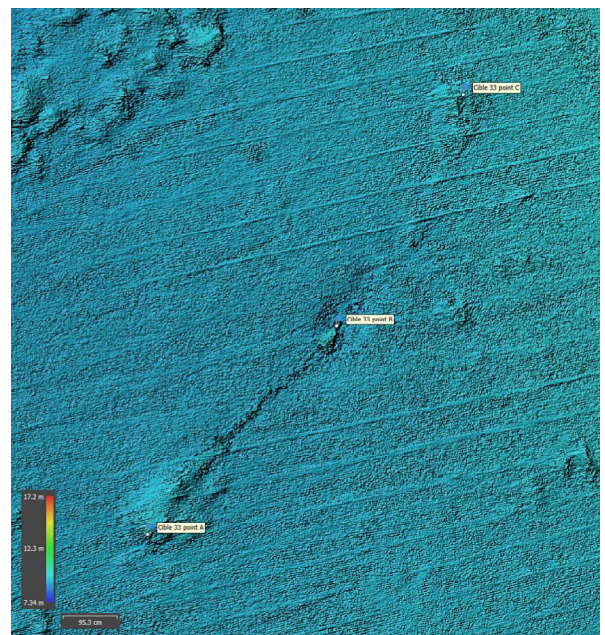
HQ SS MBES Cible 33
