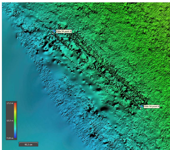
HQ SS MBES Cible 54
