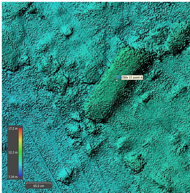
HQ SS MBES Cible 12
