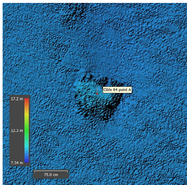
HQ SS MBES Cible 64
