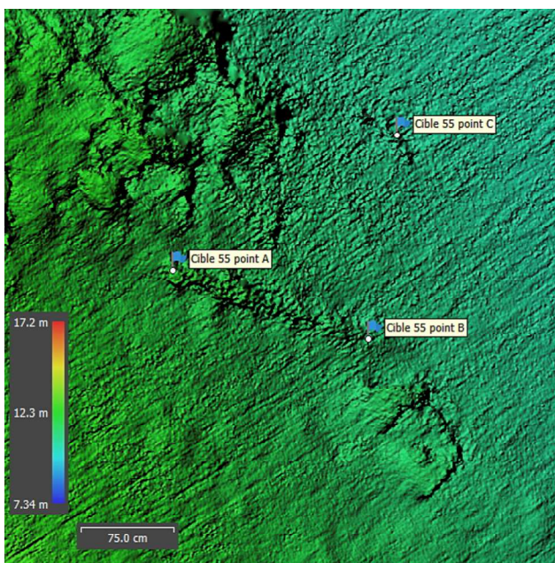
HQ SS MBES Cible 55
