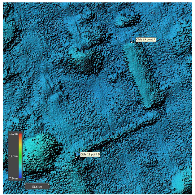
HQ SS MBES Cible 19
