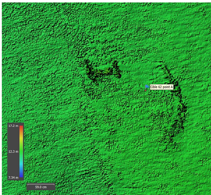
HQ SS MBES Cible 62
