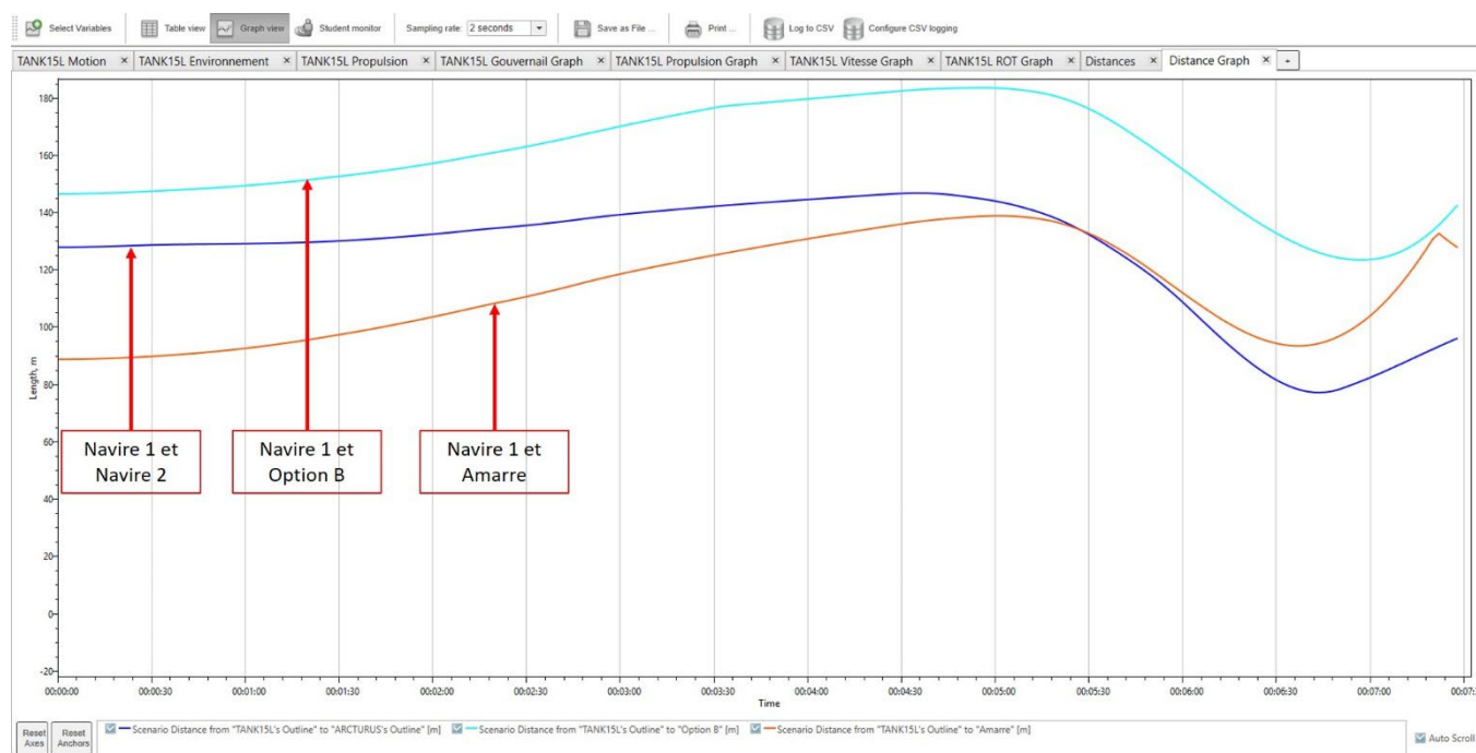
Graphique 10 (SIM 08) : distances en continu entre le navire 1 et : Le navire accosté à QSL/Le navire 1 et l'Option B/Le navire 1 et l'amarre arrière du navire accosté à QSL.
