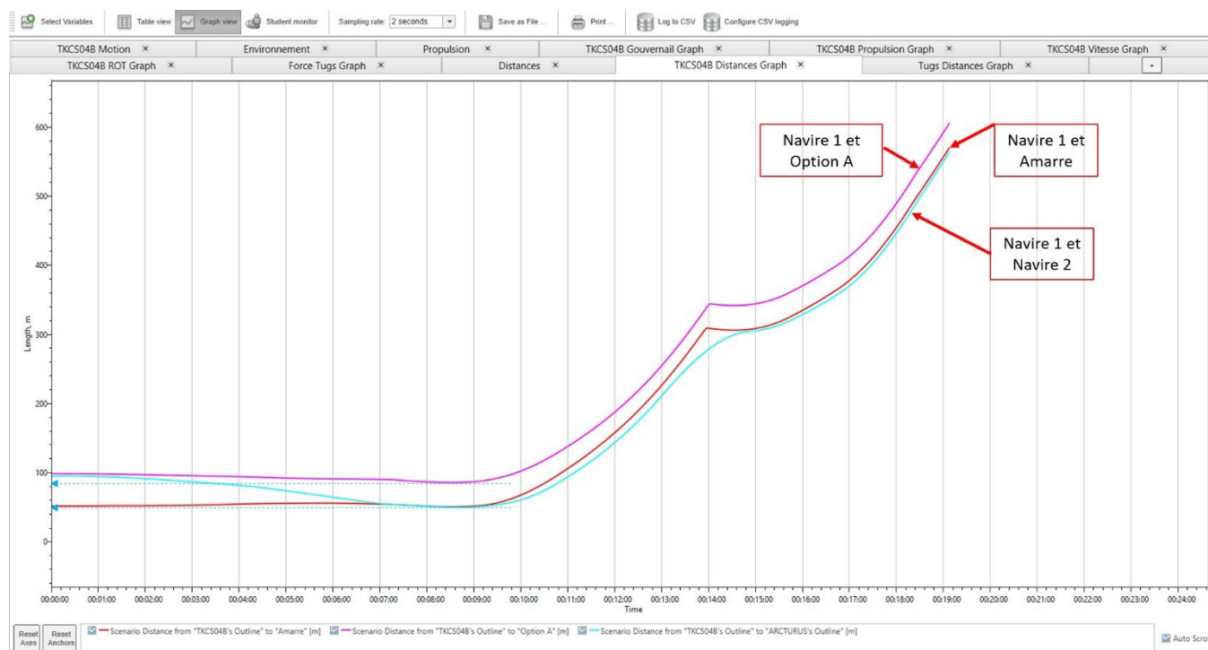
Graphique 3 (SIM 01B) : distances en continu entre le navire 1 et : L'option A/Le navire accosté à QSL/L'amarre arrière du navire accosté à QSL.
