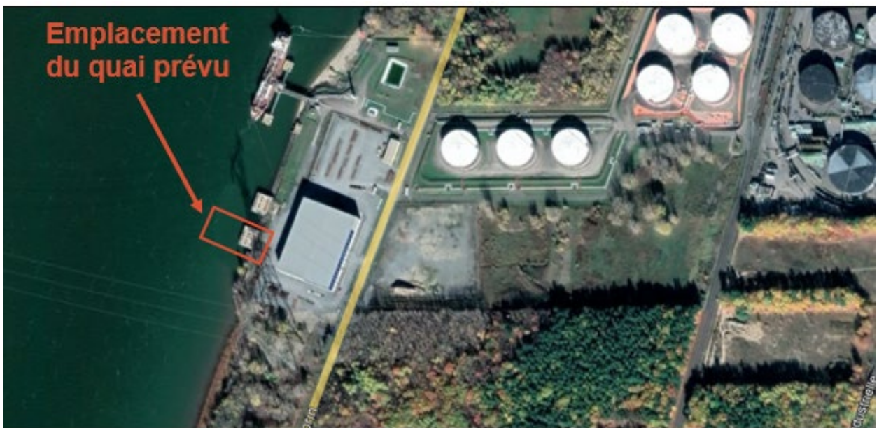
Figure 2 : Emplacement prévu du quai incluant le bâtiment d'entreposage construit
