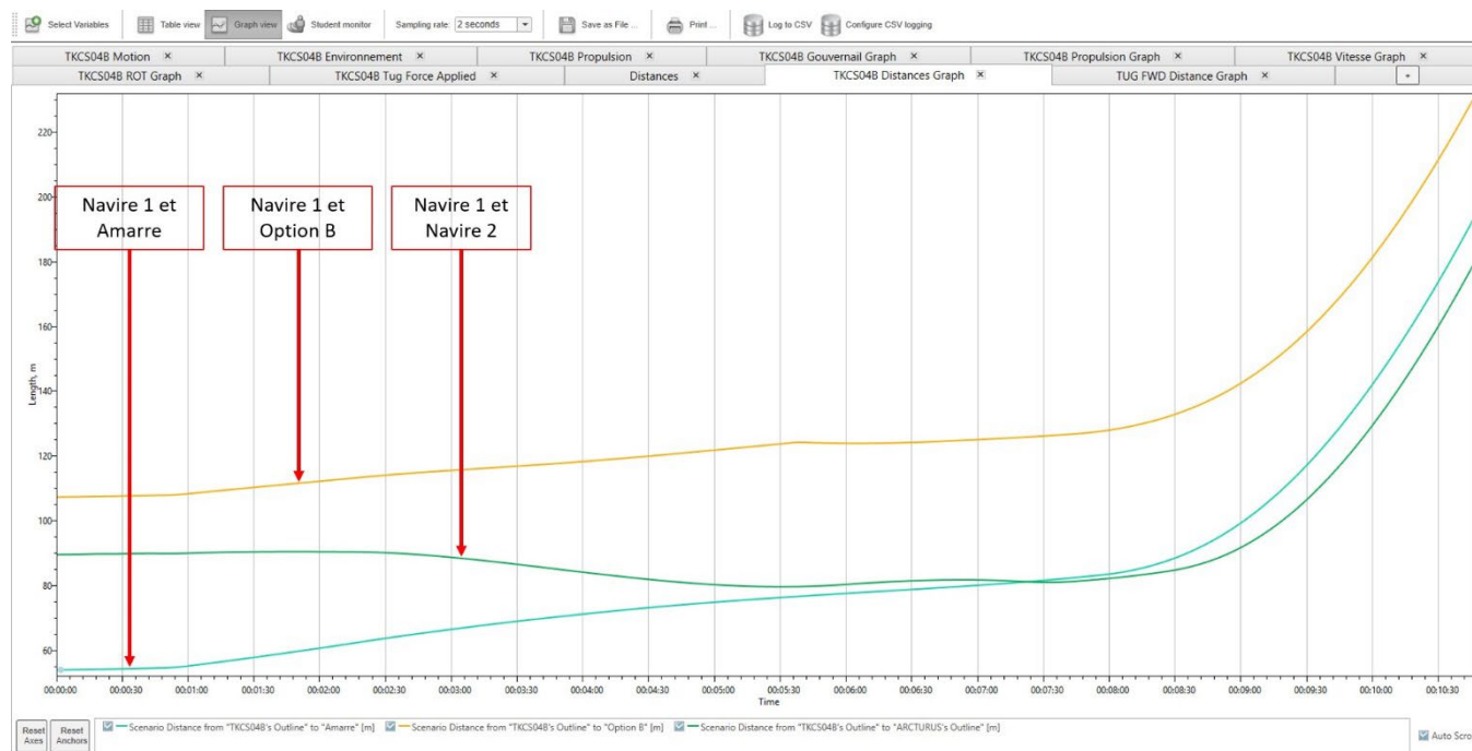
Graphique 8 (SIM 07) : distances en continu entre le navire 1 et : L'amarre arrière du navire accosté à QSL./L'option A/Le navire accosté à QSL.
