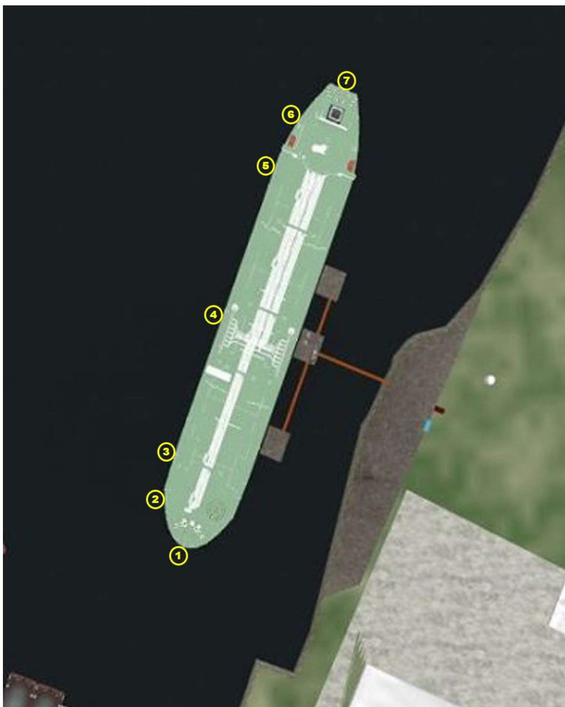
Illustration 11: Points d'attache des remorqueurs
