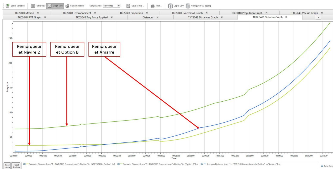
Graphique 9 (SIM 07) : distances en continu entre le navire 1 et : Le remorqueur et le navire accosté à QSL/Le remorqueur et l'Option B/Le remorqueur et l'amarre arrière du navire accosté à QSL.
