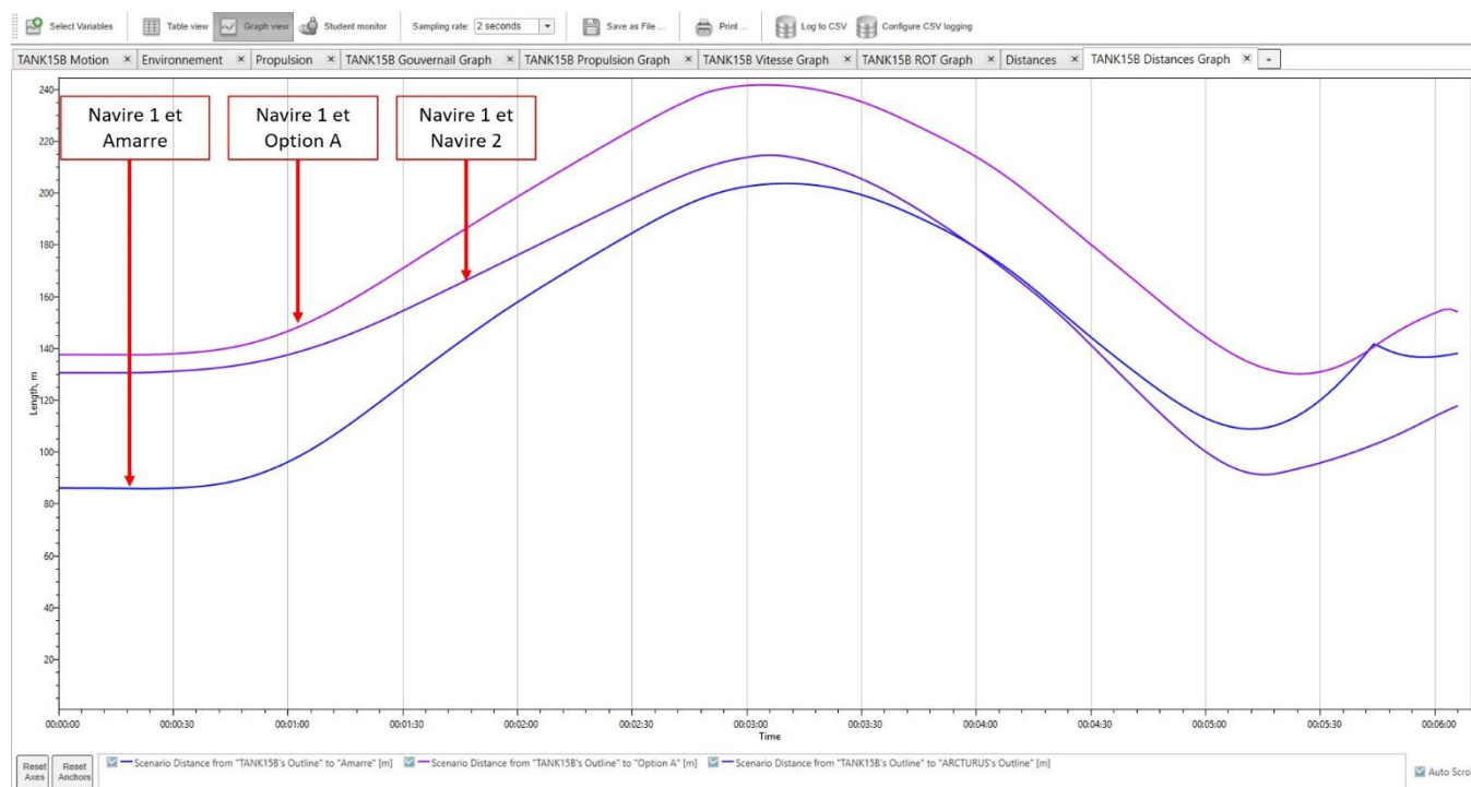
Graphique 7 (SIM 04) : distances en continu entre le navire 1 et : L'amarre arrière du navire accosté à QSL./L'option A/Le navire accosté à QSL.
