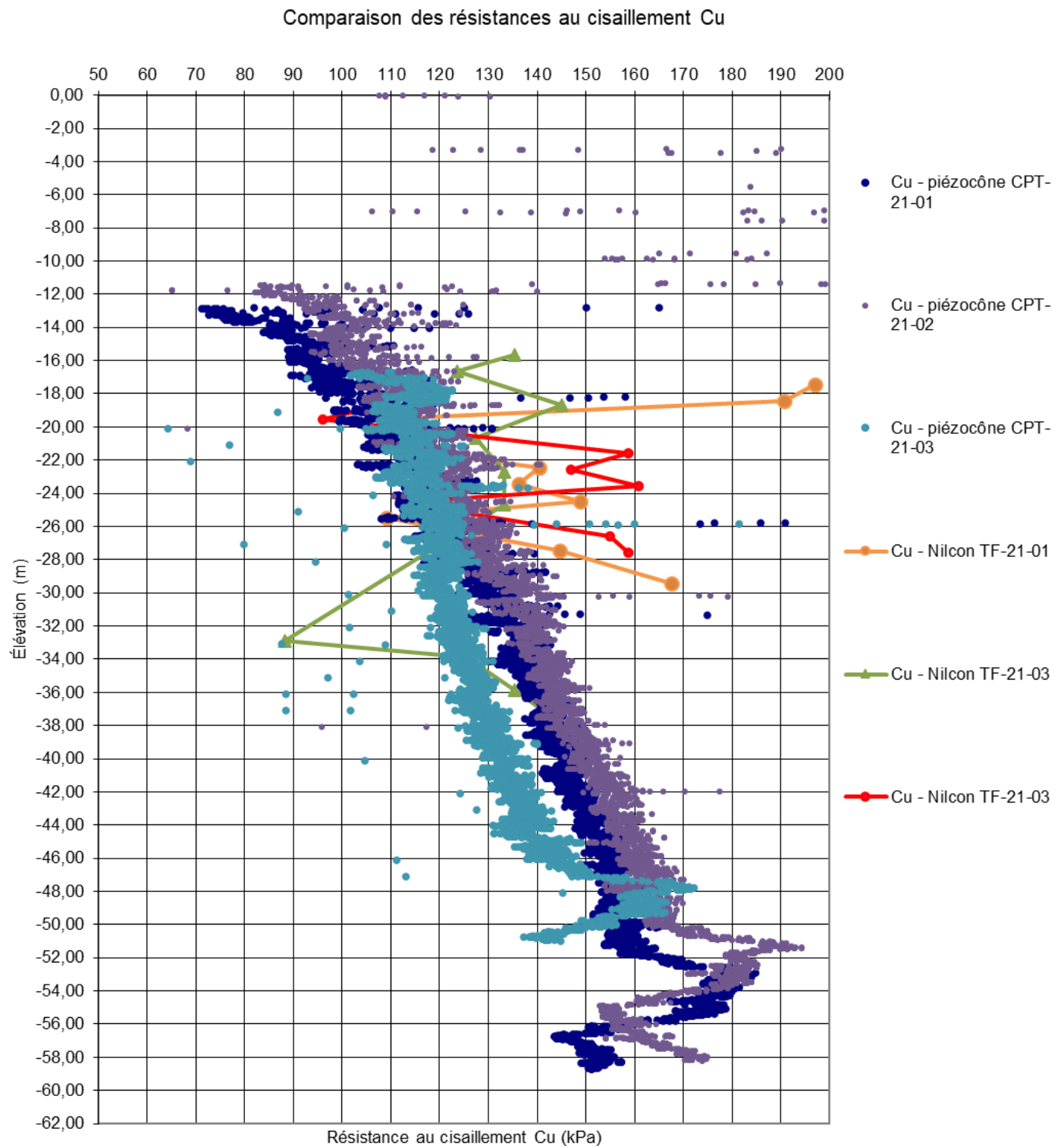
Figure 3 : Résultats des résistances au cisaillement non drainé obtenus selon les essais CPT et les valeurs des mesures au scissomètre
