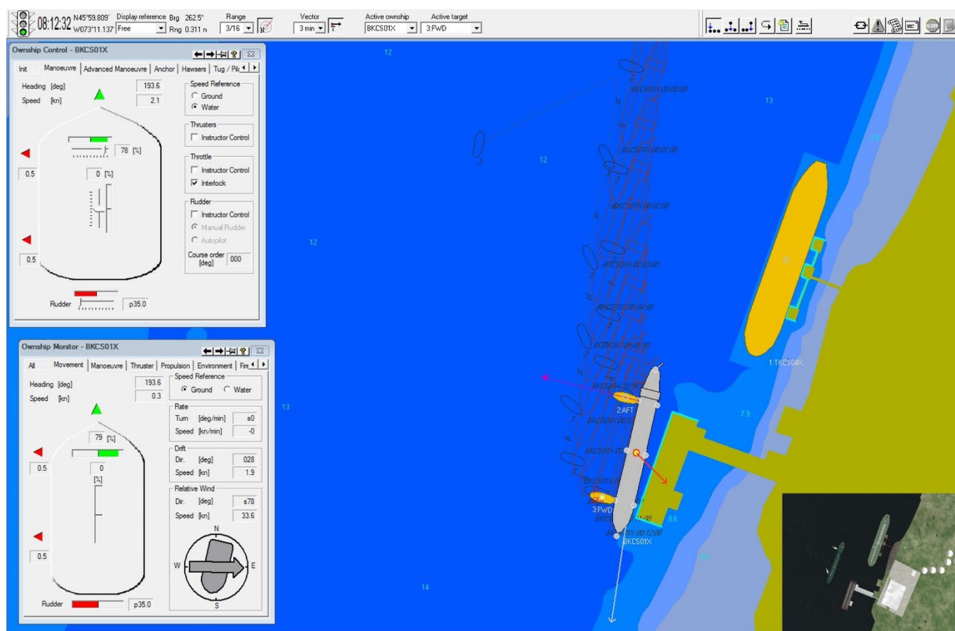
Illustration 17: Saisie d'écran de l'exercice (SIM 05).
