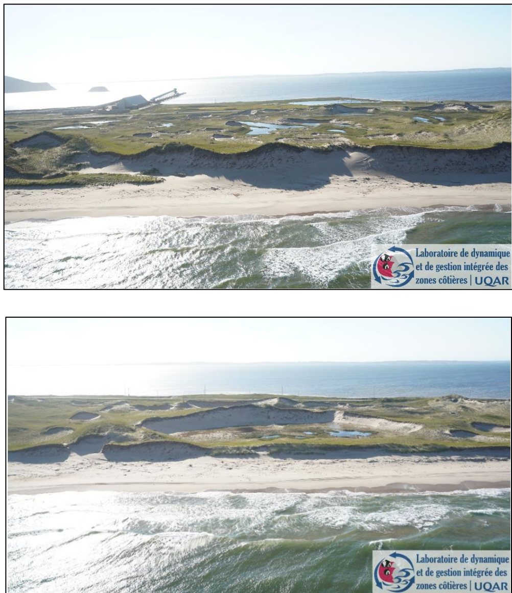
Figure 5. Photographies aériennes du secteur de Mines Seleine (septembre 2021). On distingue bien les fronts de dune en érosion ainsi que le fond des caoudères à de basses altitudes.
