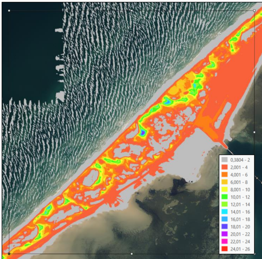
Figure 6. Topographie (élévation en mètres). On observe que plusieurs caoudères sont situés près du front de dune en érosion et qu'environ 20% du territoire a une altitude inférieure à 2 m.
