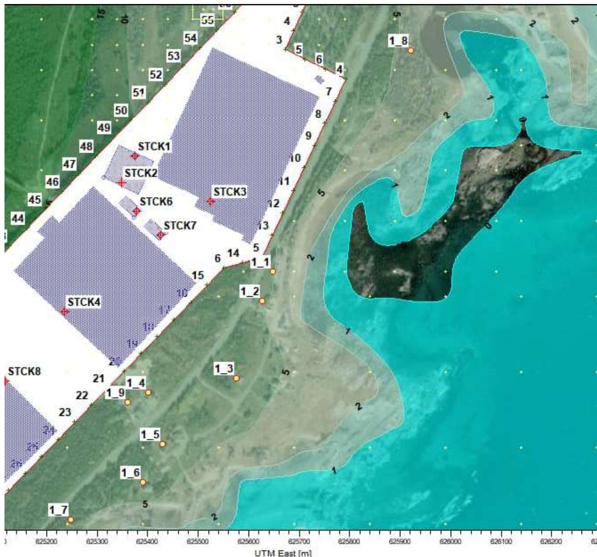
Figure 5 : Vue des récepteurs couvrant la zone (image tirée du logiciel ISC-AERMOD View)
