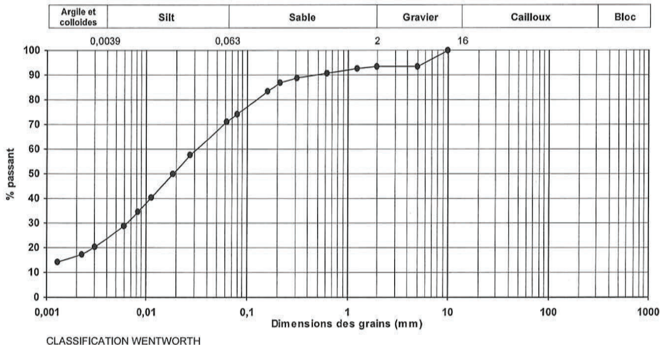
Courbe granulométrique
