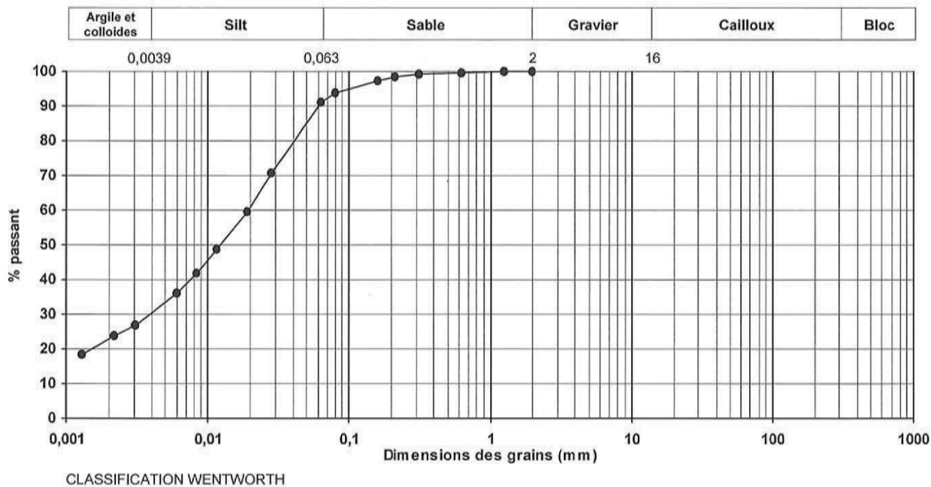
Courbe granulométrique
