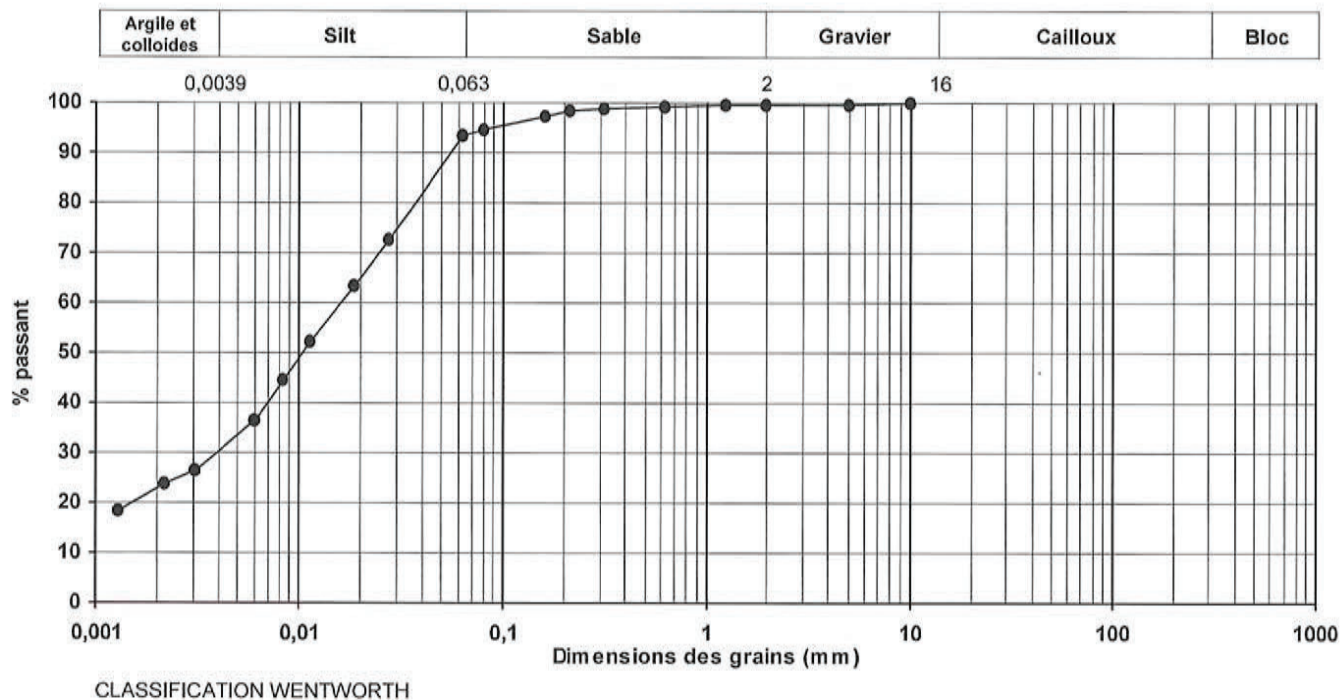
Courbe granulométrique
