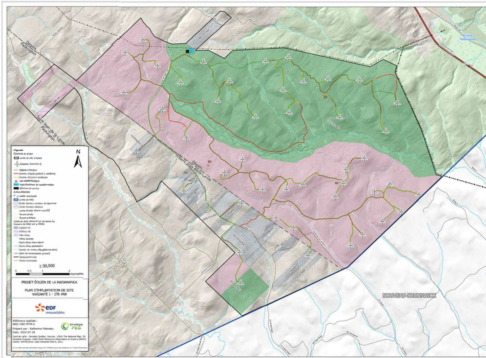
Figure A-1 - Plan d'implantation du parc éolien
