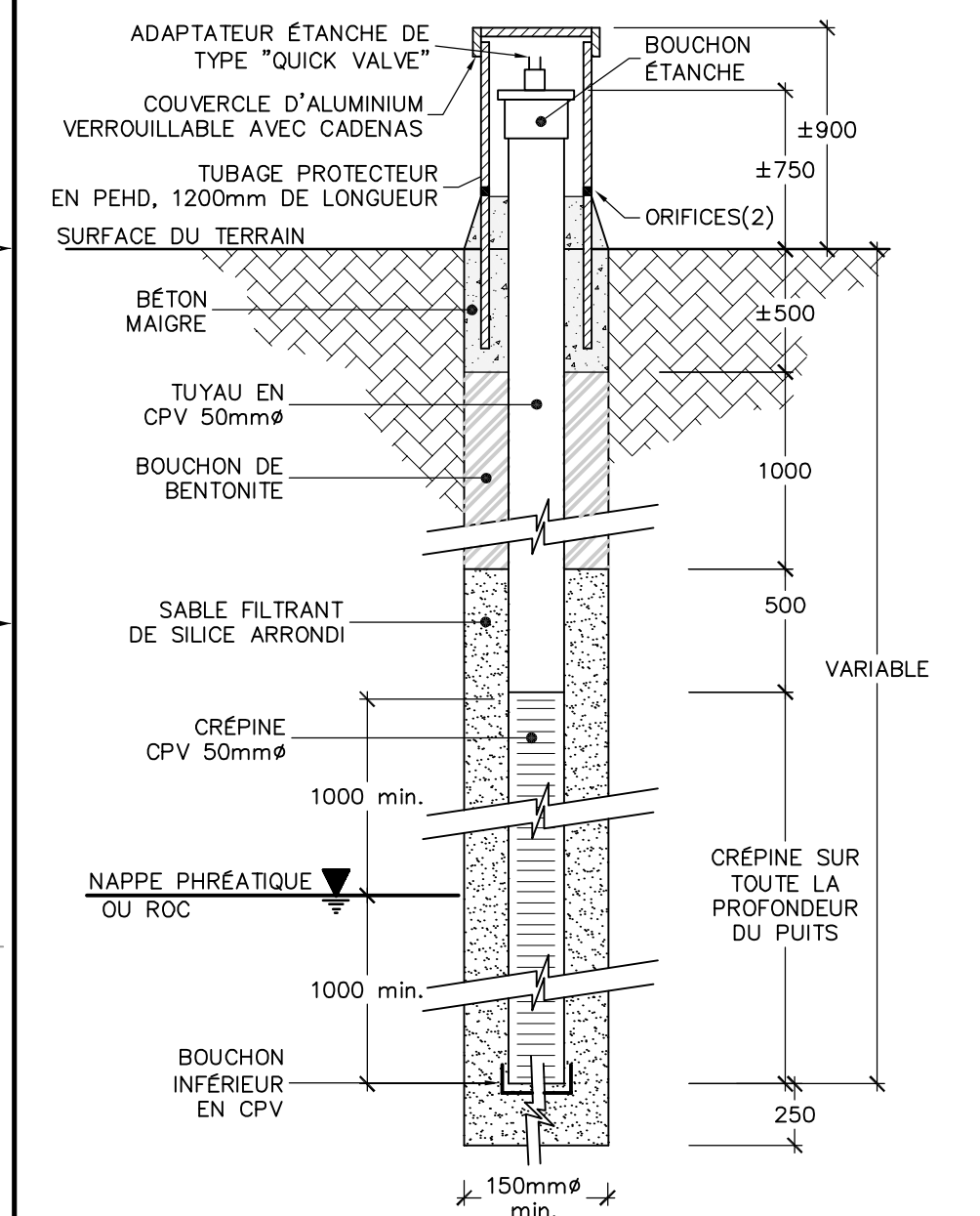
121254-1 PUITS D'OBSERVATION (SB) DES BIOGAZ TYPIQUE Échelle: aucune
