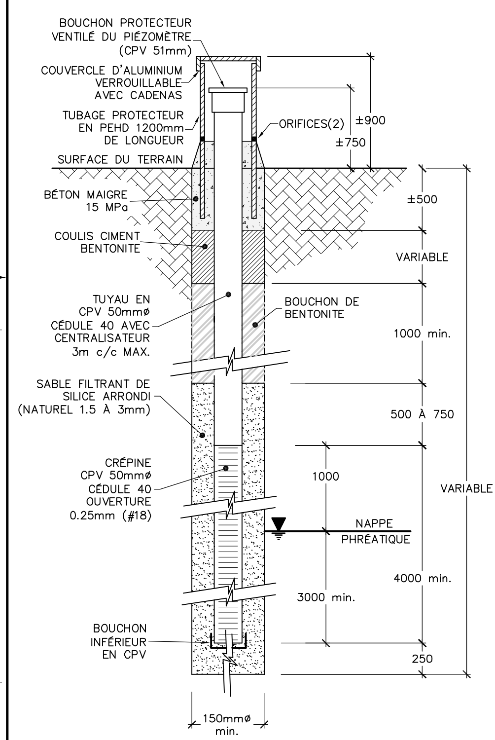
121253-1 PUITS D'OBSERVATION (PO) DES EAUX SOUTERRAINES TYPIQUE Échelle: aucune
