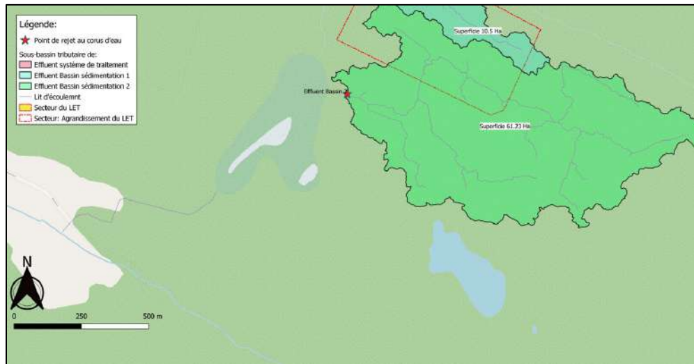
Figure 3-3 : Sous-bassin tributaire de l'effluent du bassin de sédimentation 2 (BS-5)
