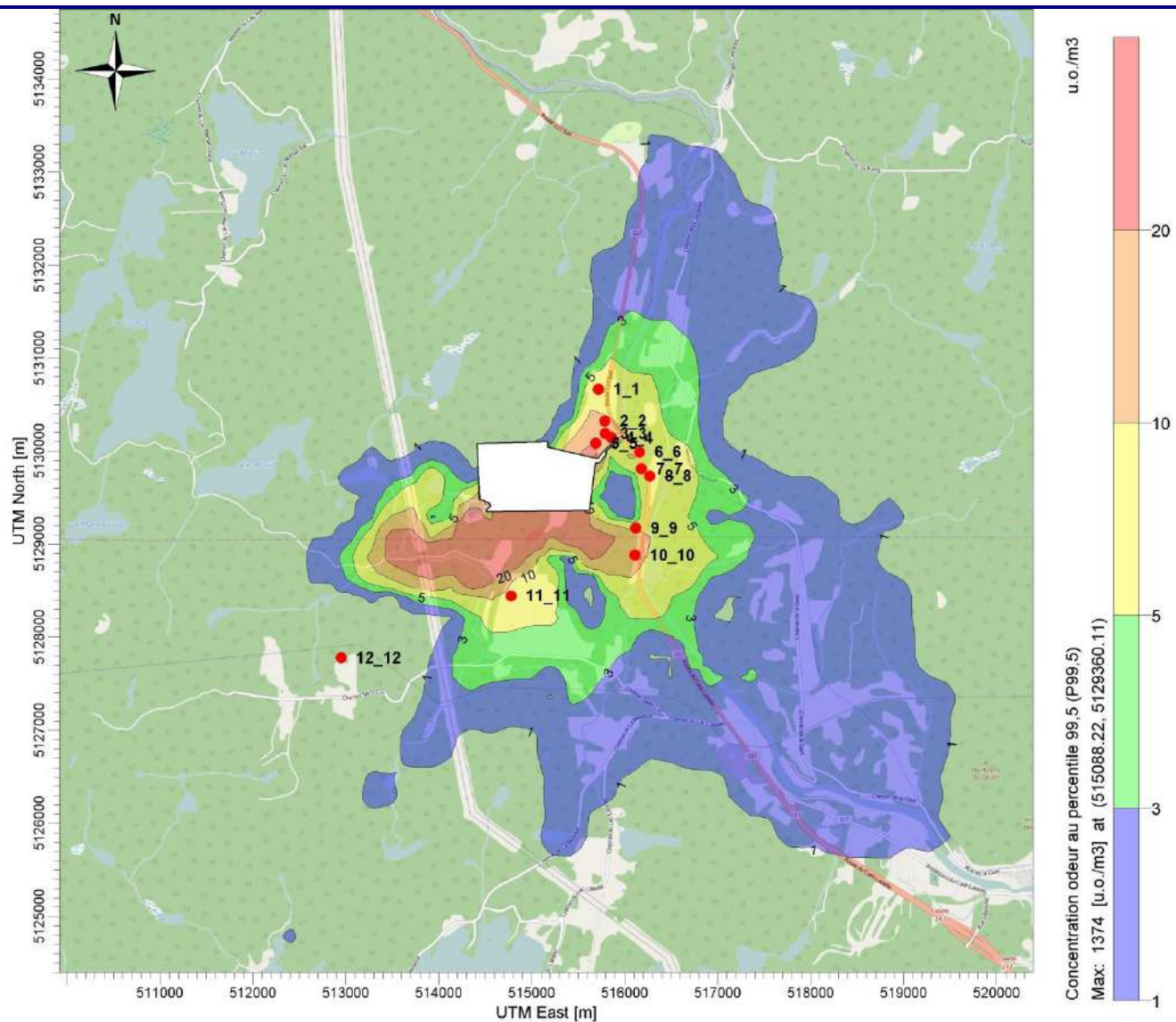
Figure H-2 : Concentration odeur P99,5 - Scénario 1
