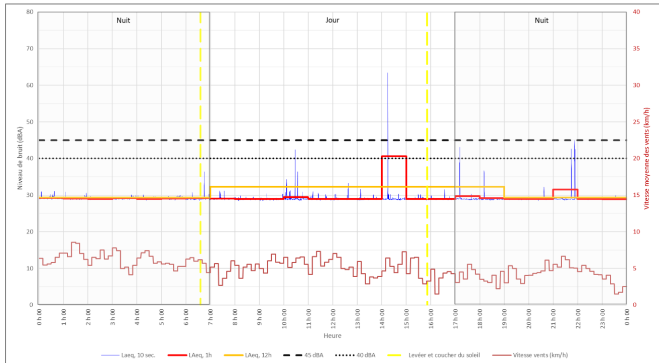
Figure A4.5 : Évolution temporelle du bruit enregistrée au point P3 (8 e Rang) le 13 novembre 2023.
