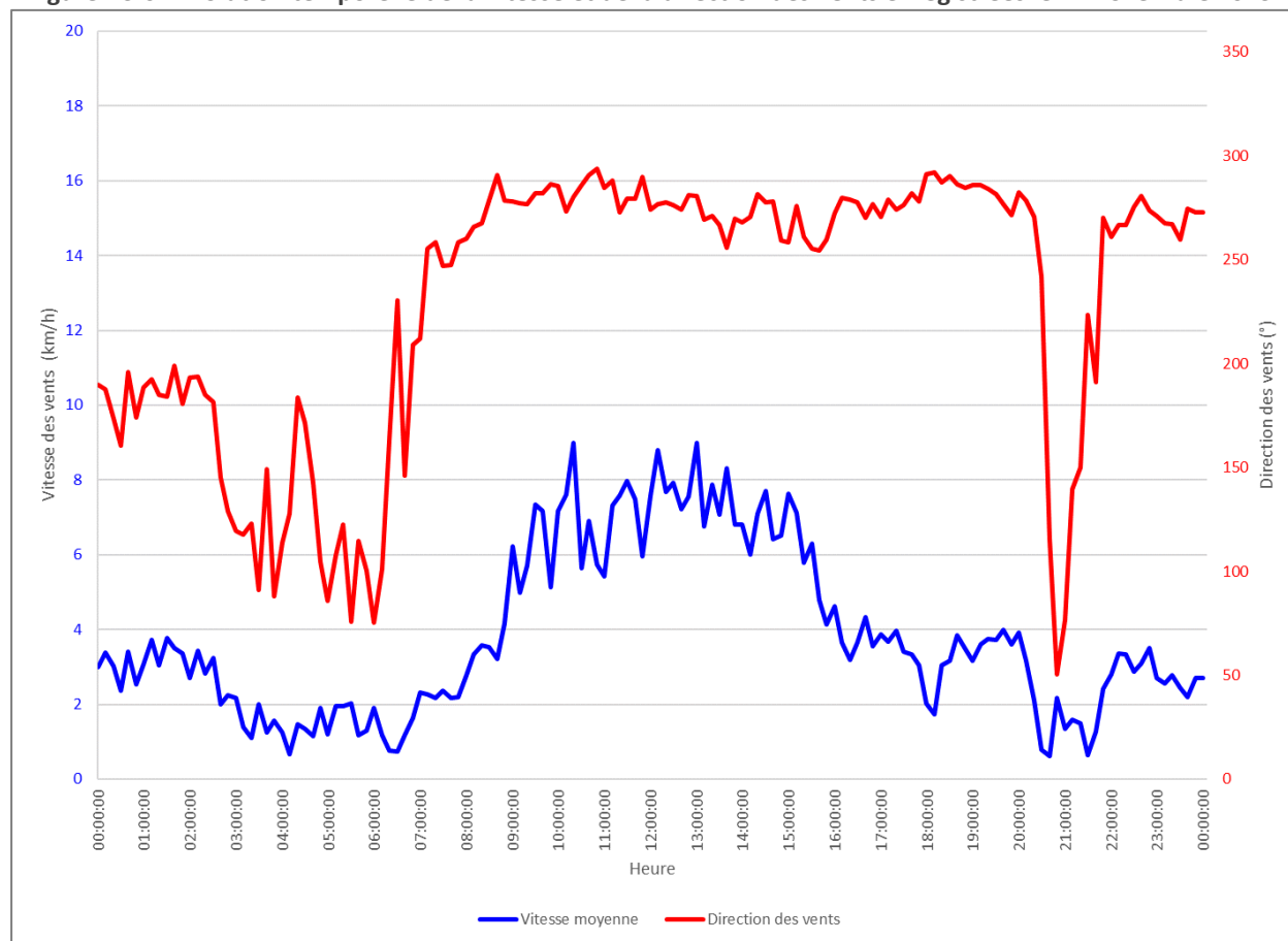
Figure A3.6 : Évolution temporelle de la vitesse et de la direction des vents enregistrées le 14 novembre 2023.
