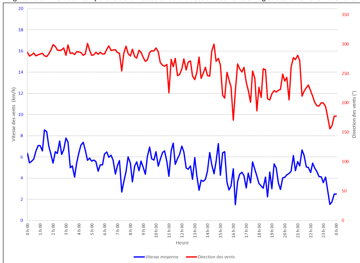
Figure A3.3 : Évolution temporelle de la vitesse et de la direction des vents enregistrées le 13 novembre 2023.
