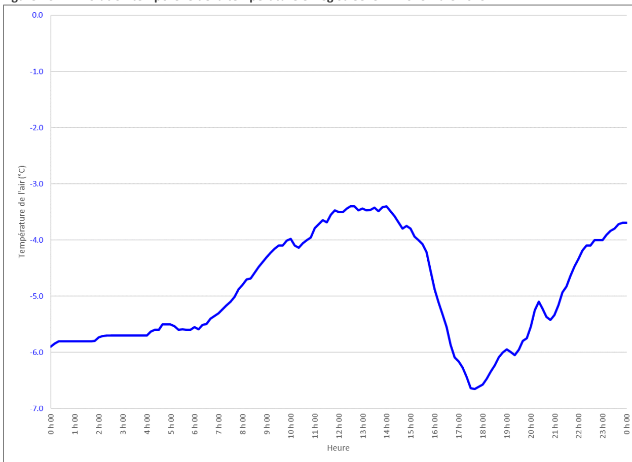
Figure A3.4 : Évolution temporelle de la température enregistrée le 14 novembre 2023.
