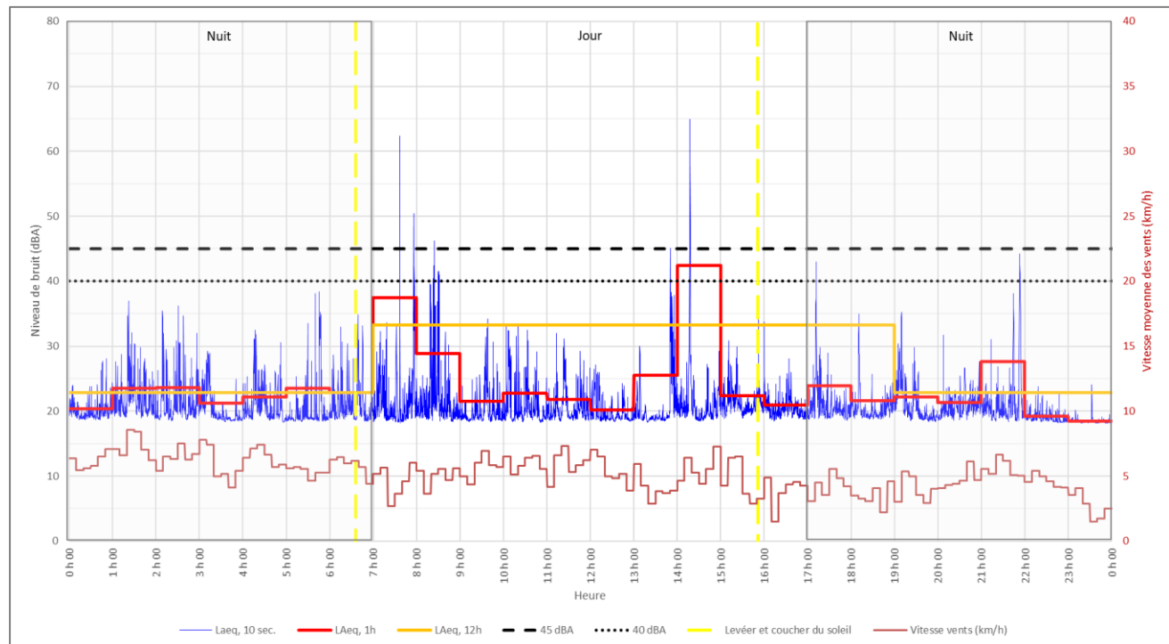
Figure A4.1 : Évolution temporelle du bruit enregistrée au point P1 (10 e Rang) le 13 novembre 2023.
