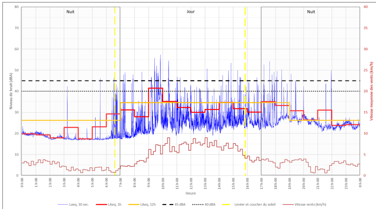
Figure A4.4 : Évolution temporelle du bruit enregistrée au point P2 (8 e Rang) le 14 novembre 2023.
