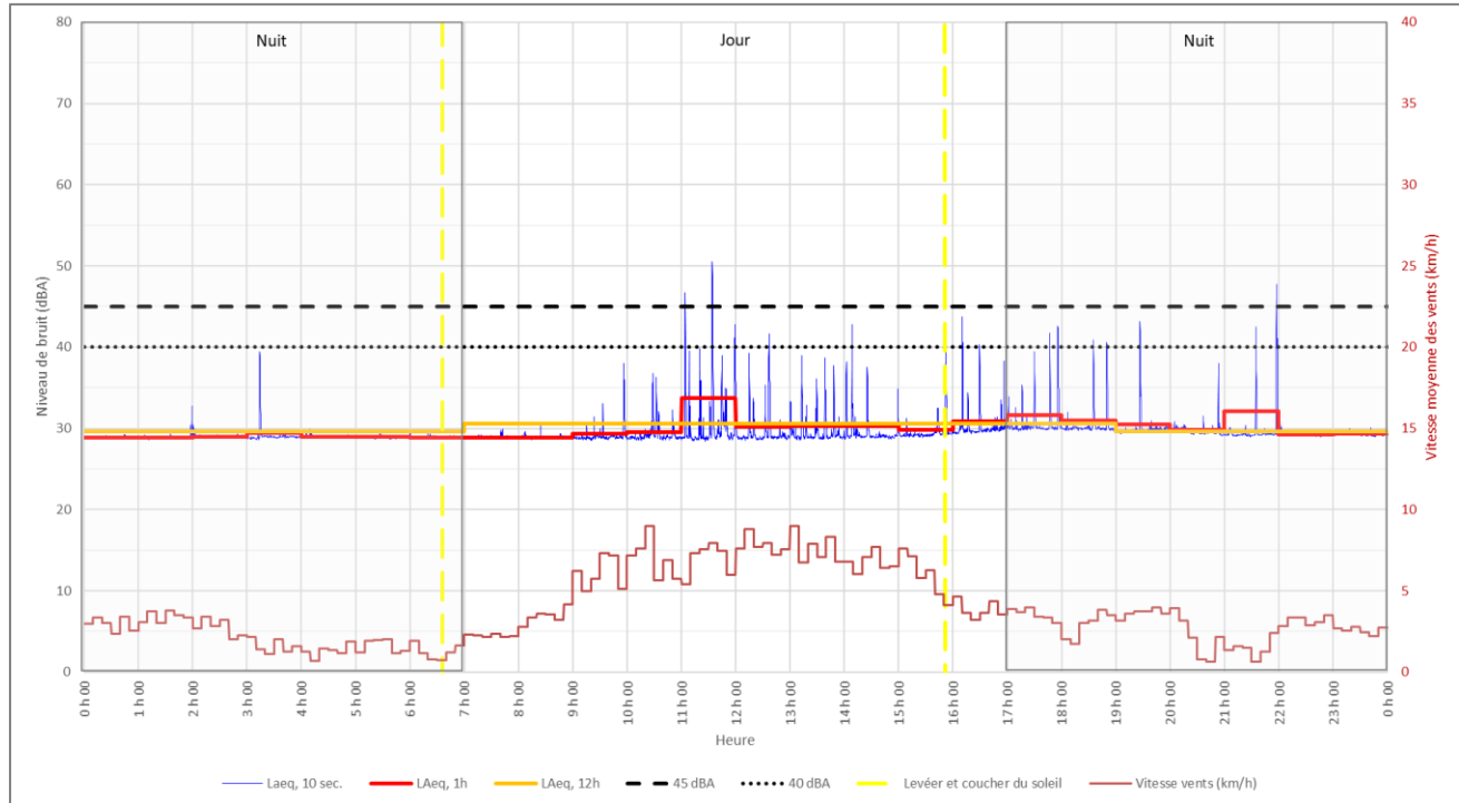
Figure A4.6 : Évolution temporelle du bruit enregistrée au point P3 (8 e Rang) le 14 novembre 2023.
