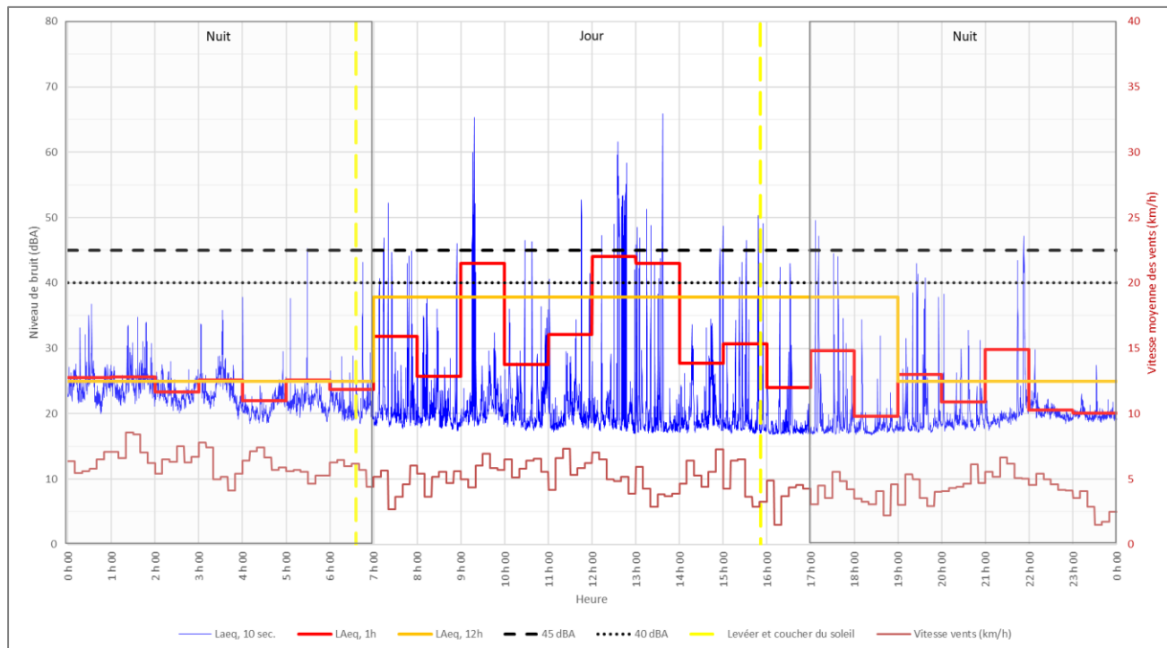
Figure A4.3 : Évolution temporelle du bruit enregistrée au point P2 (8 e Rang) le 13 novembre 2023.
