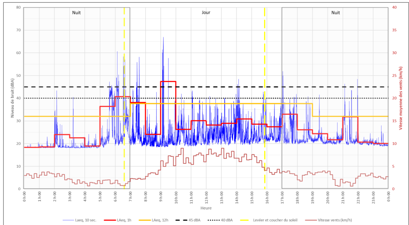
Figure A4.2 : Évolution temporelle du bruit enregistrée au point P1 (10 e Rang) le 14 novembre 2023.
