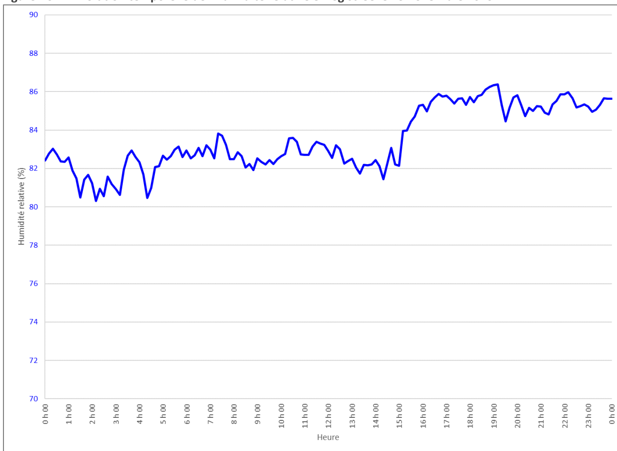
Figure A3.2 : Évolution temporelle de l'humidité relative enregistrée le 13 novembre 2023.
