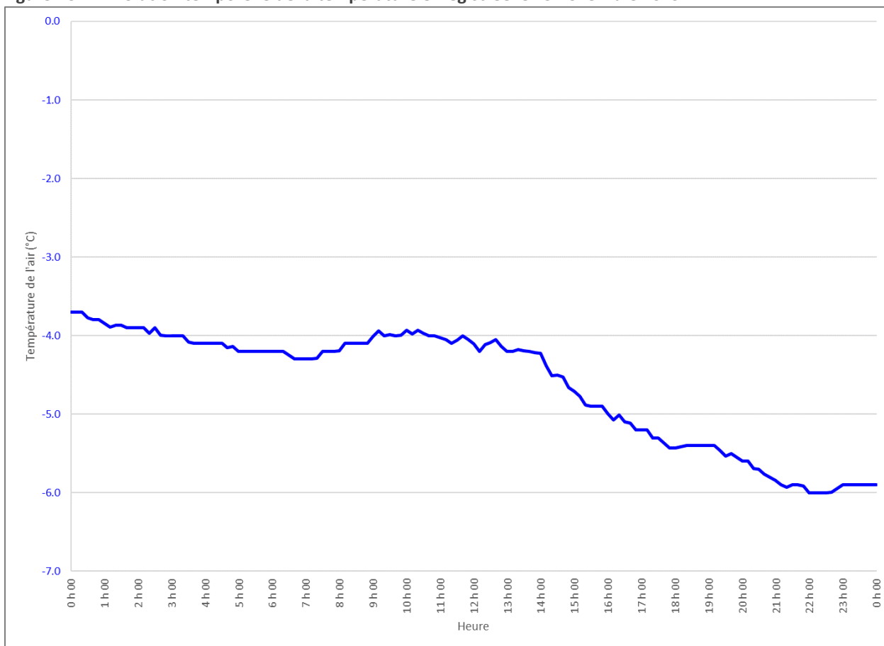
Figure A3.1 : Évolution temporelle de la température enregistrée le 13 novembre 2023.
