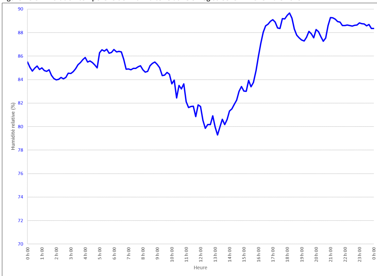
Figure A3.5 : Évolution temporelle de l'humidité relative enregistrée le 14 novembre 2023.
