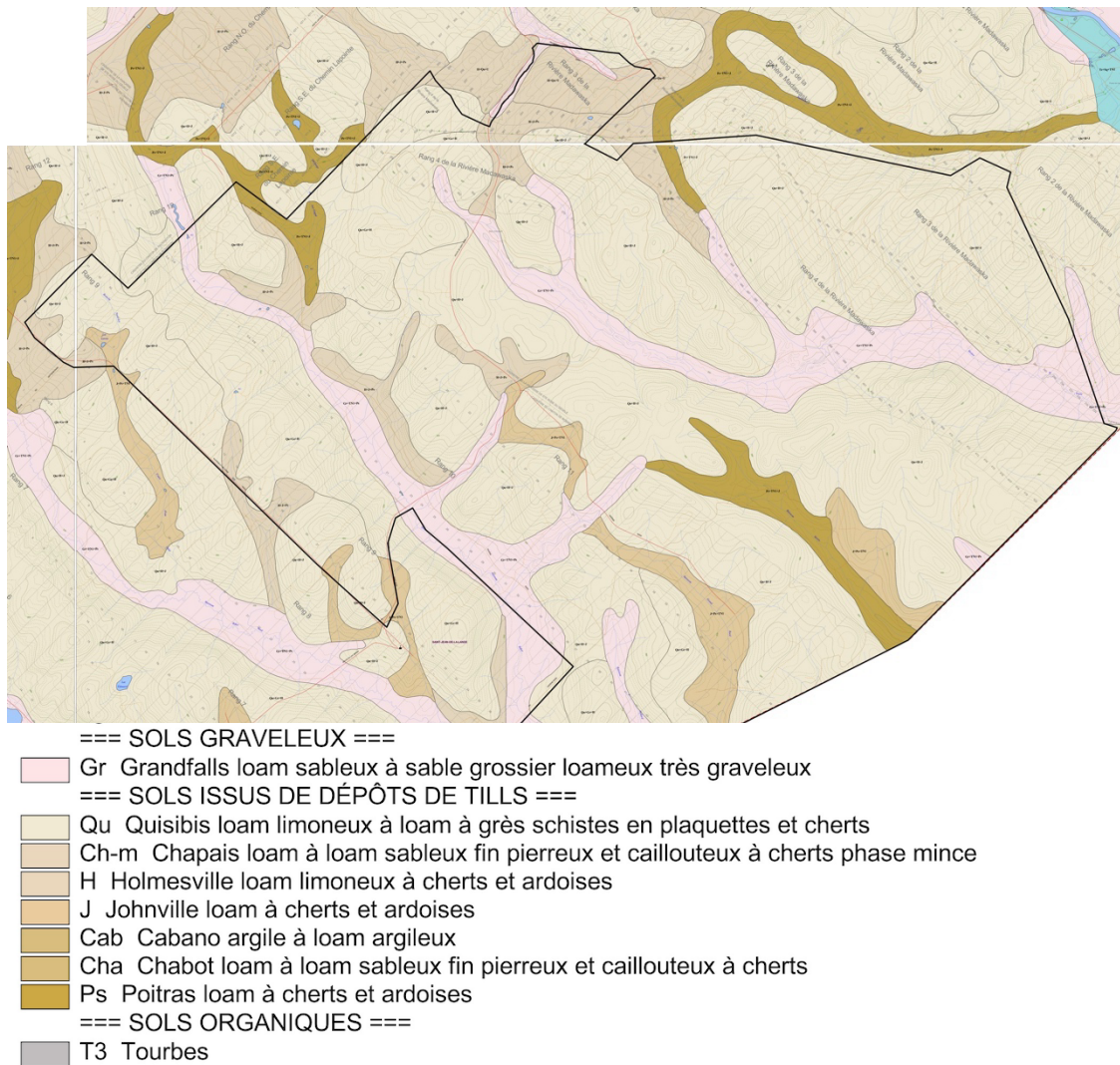
Figure 8 Pédologie des sols du secteur à l'étude (IRDA, 21N07, 21N10)
