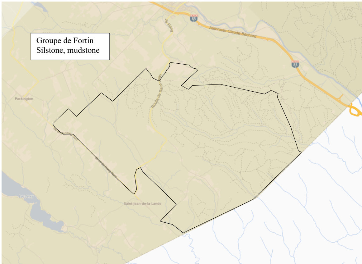
Figure 6 Géologie du secteur à l'étude (Sigeom interactif 2023)
