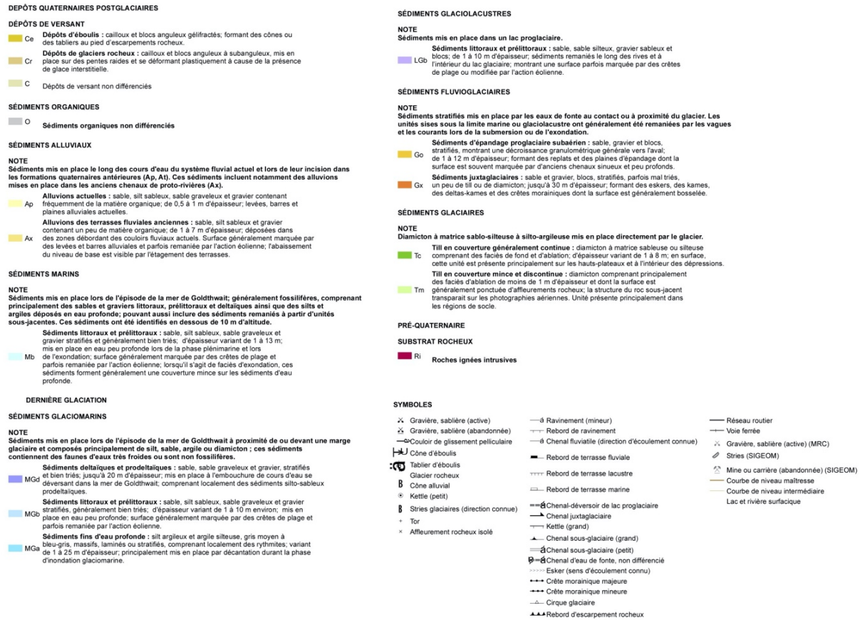
Figure 5 Dépôts de surface du quaternaire du secteur à l'étude, légende (DDEFPPQ, 2014, 21M07 et 21M10)
