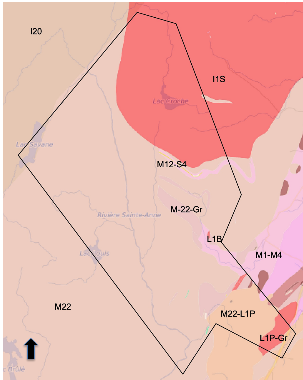
Figure 4 Géologie du secteur à l'étude (Sigeom interactif 2021)
