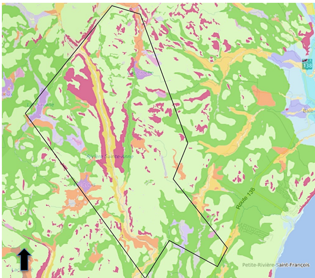
Figure 5 Dépôts de surface du quaternaire du secteur à l'étude (Sigeom interactif 2021)
