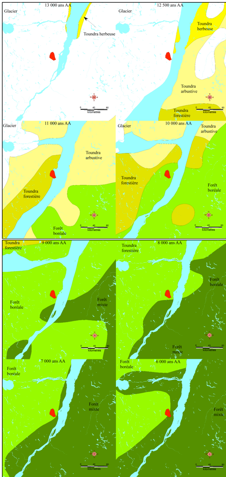
Figure 8 Les principales étapes de la déglaciation et de l'évolution de la végétation (le secteur à l'étude est représenté par le polygone rouge au centre) (Dyke et coll. 2004)
