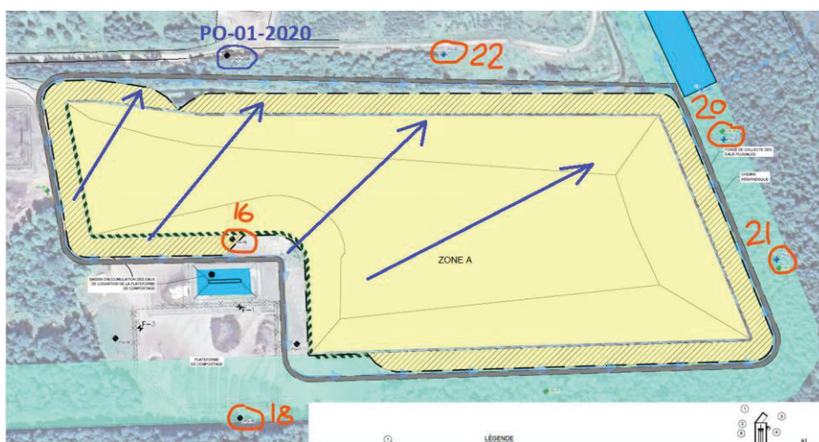
Figure 2 : Représentation de l'écoulement radial. Adapté du dessin 43955TT-ENV-SE01 (TetraTech, 2023-12-13).
