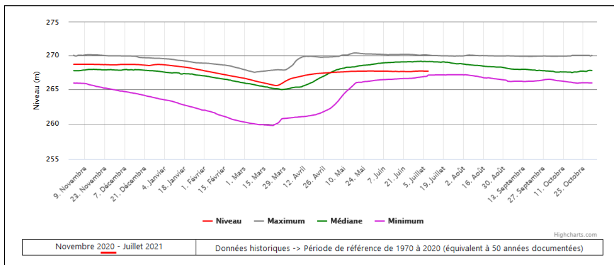
Figure 2 Niveau d'eau à la station : 040608 Barrage Kiamika
