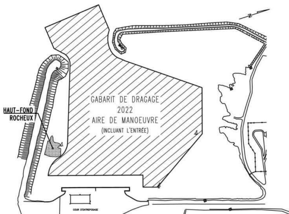
Figure 14 - Gabarit de dragage – 2022 - Aire de manœuvre
