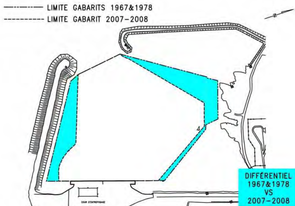
Figure 12 - Gabarits de dragage – Comparaison - 2007-2008 vs 1967 & 1978
