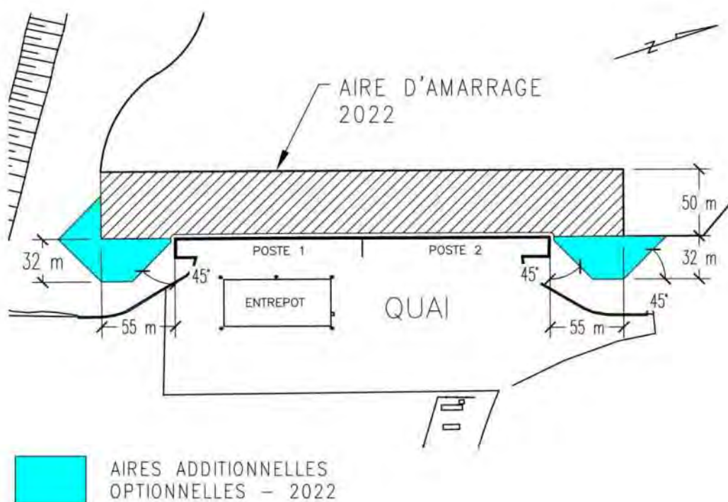
Figure 15 – Gabarit de dragage – 2022 - Aire d'amarrage et Aires additionnelles
