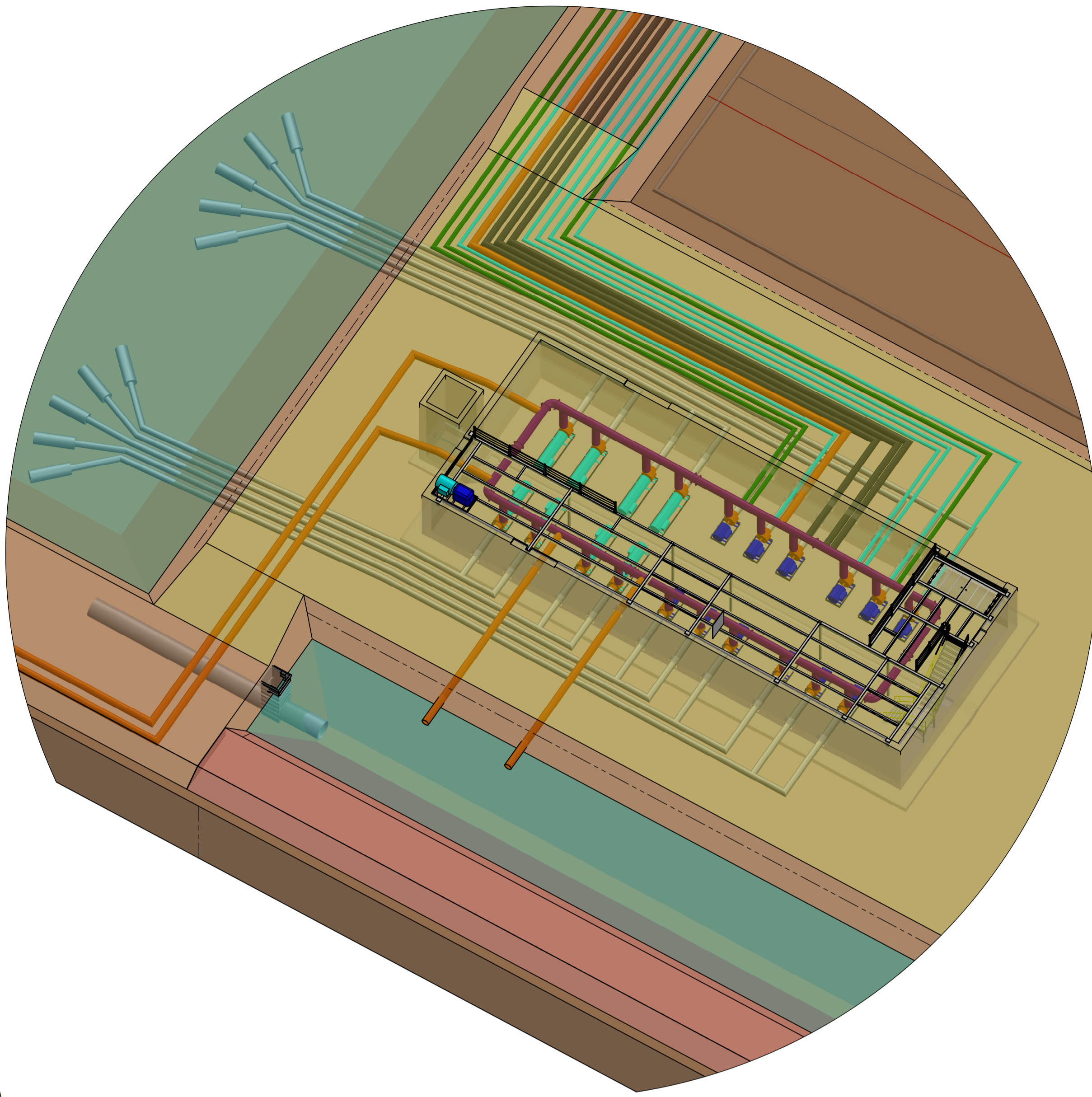
VUE ISOMETRIQUE - BÂTIMENT DES POMPES -
