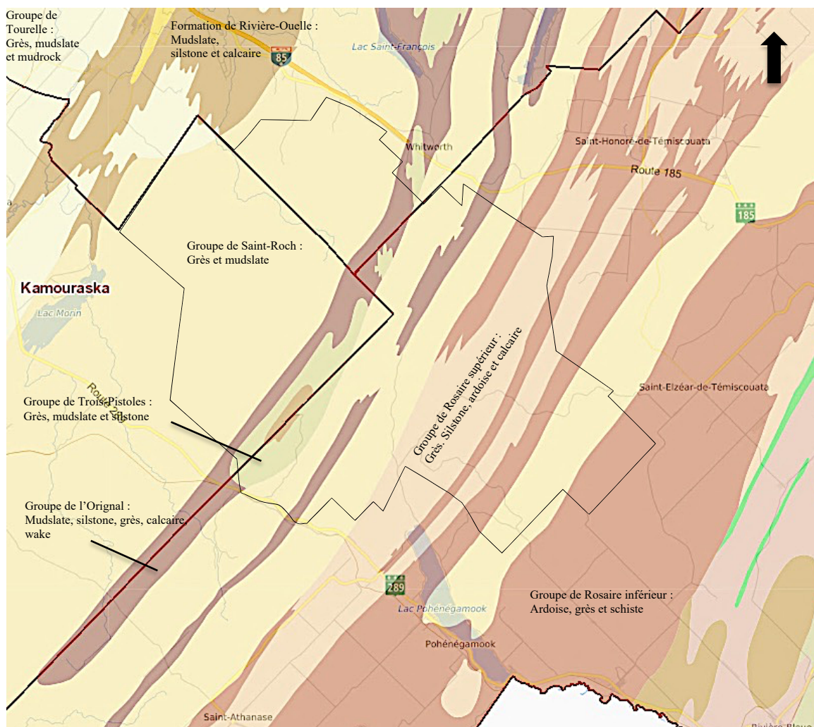
Figure 6 Géologie du secteur à l'étude (Sigeom interactif 2022)
