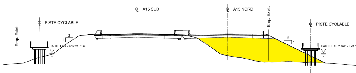
Figure 2-31 Coupe de la jetée de l'approche sud
