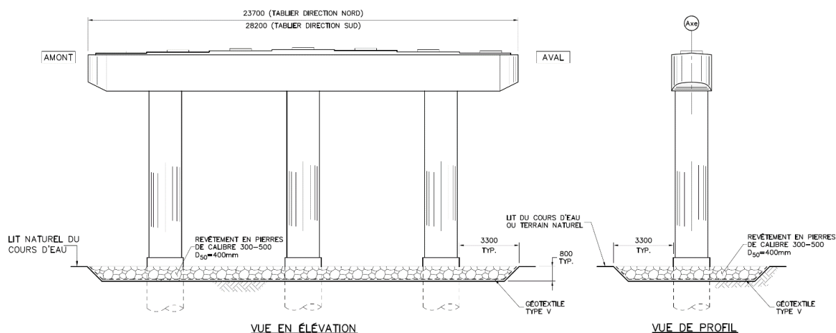
Figure 2-7 Coupes en élévation et en profil de l'enrochement de protection des piles
