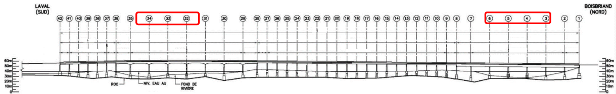
Figure 2-34 Unité de fondations du pont existant démolies à partir de barges
