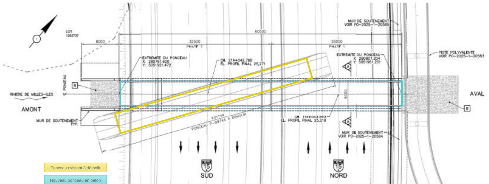
Figure 2-17 Longueur et orientation du nouveau ponceau dans la jetée sud
