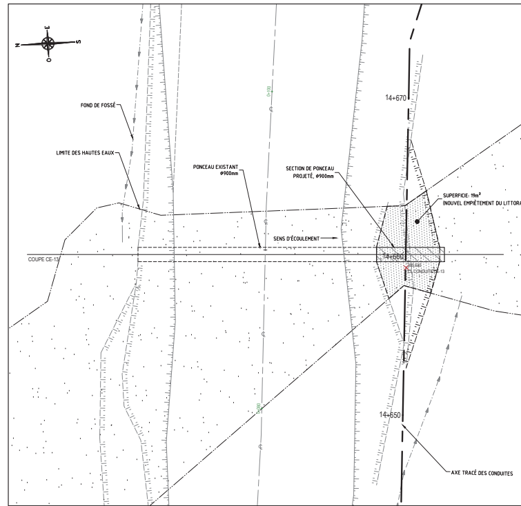
VUE EN PLAN ECH: 1/100
