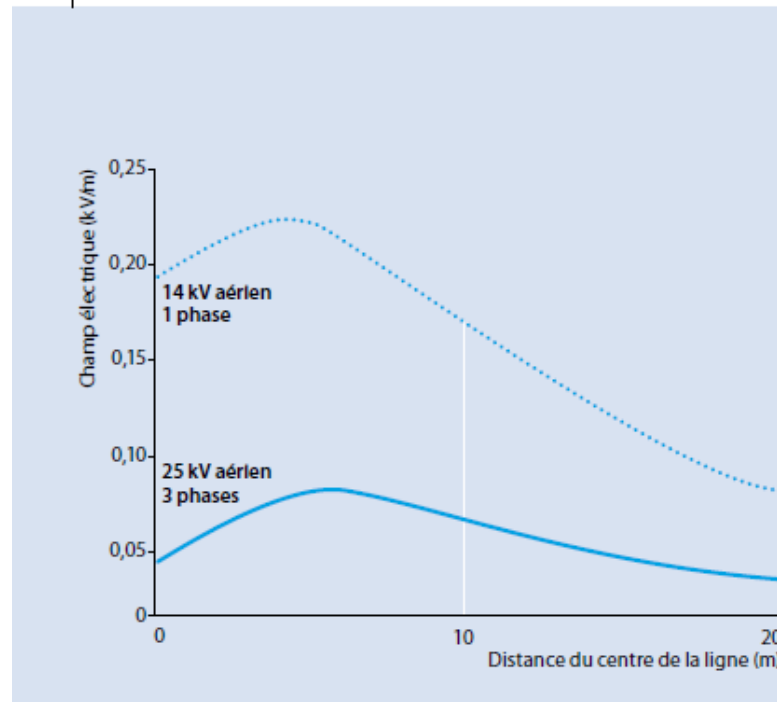
CHAMP ÉLECTRIQUE GÉNÉRÉ PAR LES LIGNES DE DISTRIBUTION (kV/m)
