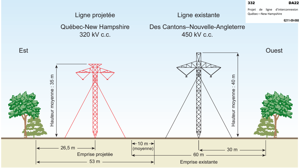
Pylônes haubanés
