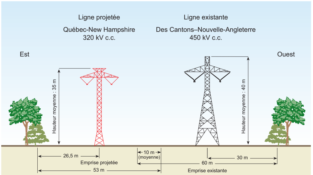
Pylônes rigides
