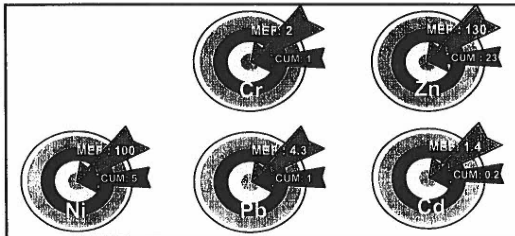
FIGURE 4.2 - RESPECT DES CRITÈRES DE PROTECTION (MEF) DANS LE MILIEU RÉCEPTEUR À 300 m DE L'EFFLUENT (CUM) EN 1996-EXPRIMÉ EN \mu\text{g/L}
