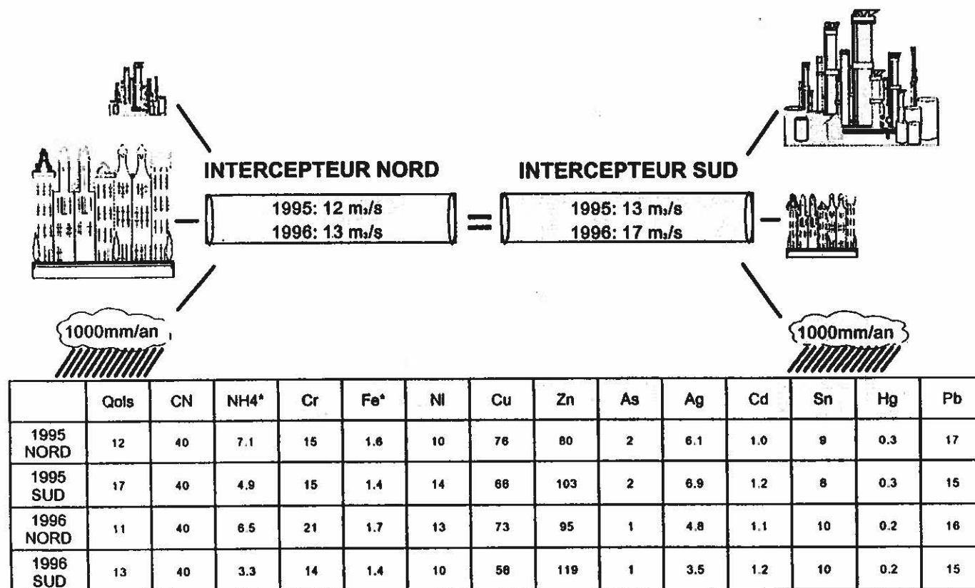
FIGURE 3.3- COMPARAISON DES CONCENTRATIONS MOYENNES ANNUELLES DANS LES EAUX BRUTES EN PROVENANCE DES DEUX INTERCEPTEURS EN 1995 ET EN 1996
