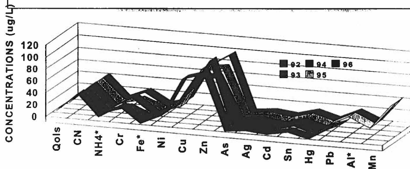
FIGURE 3.1- ÉVOLUTION DES TENEURS EN CONTAMINANTS DANS L'INTERCEPTEUR NORD DE 1992 à 1996
