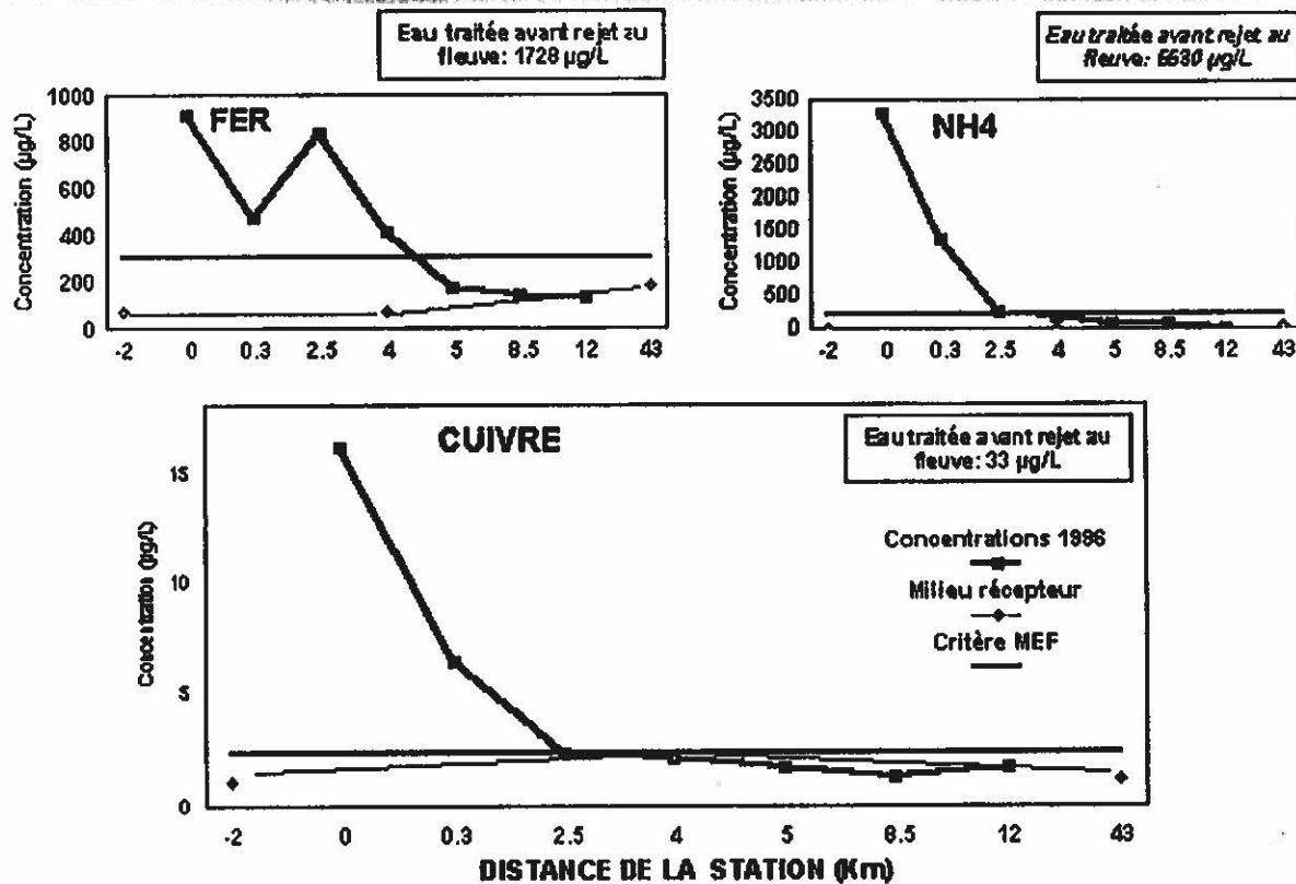
Figure 4.3 - ÉVOLUTION DES CONCENTRATIONS MESURÉES DEPUIS LA STATION D'ÉPURATION JUSQUE DANS LE MILIEU RÉCEPTEUR EN 1996 CONCENTRATIONS MOYENNES ANNUELLES
