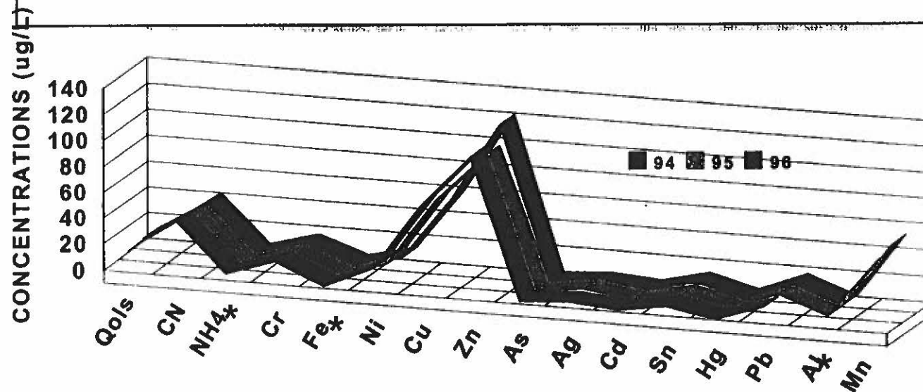
FIGURE 3.2- ÉVOLUTION DES TENEURS EN CONTAMINANTS DANS L'INTERCEPTEUR SUD DE 1994 à 1996
