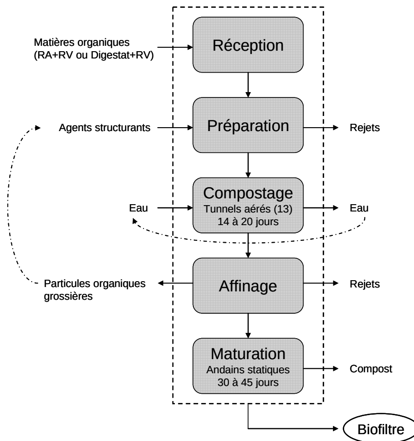
Figure 5.5 Schéma simplifié du concept de compostage en système fermé
