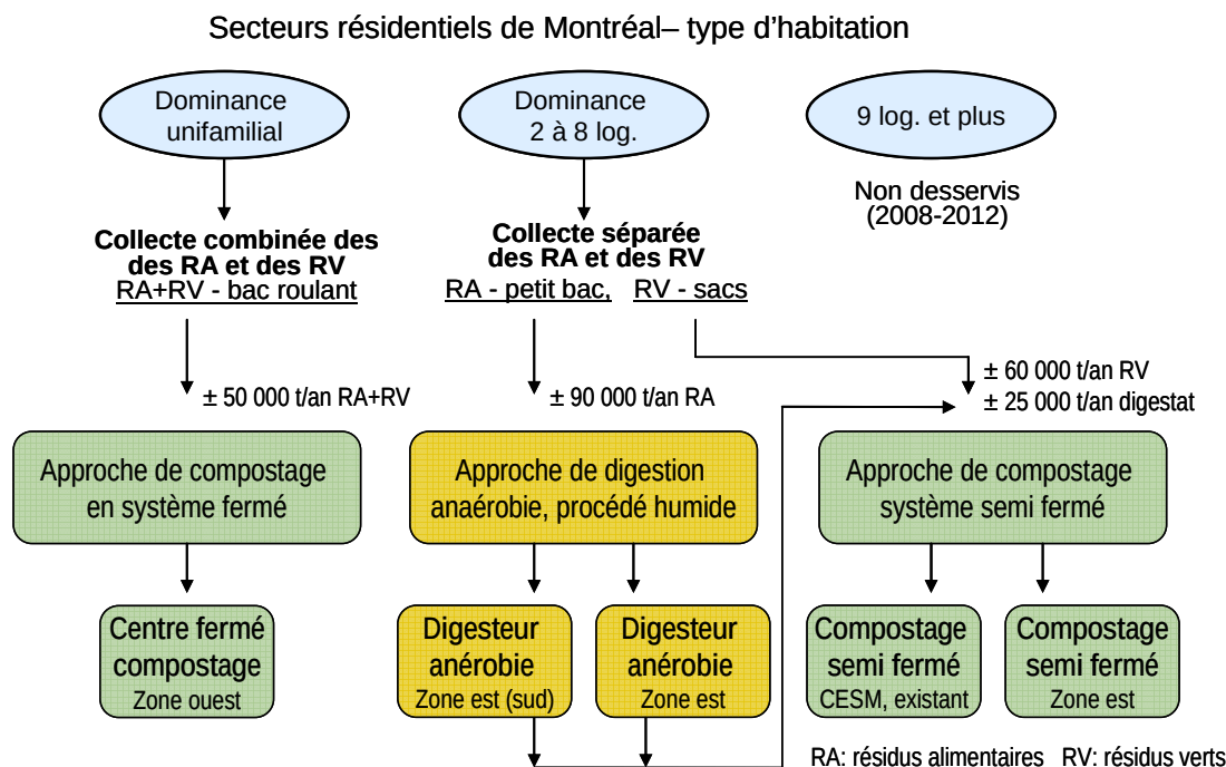
Figure 2.1 Agencement de base des installations de traitement des matières organiques requises pour Montréal, dans une perspective d'autonomie complète et en fonction des modes de collecte et des technologies privilégiées au PDGMR
