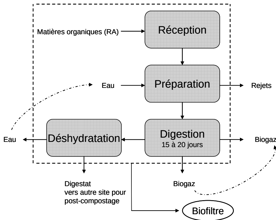
Figure 5.7 Schéma simplifié du concept de digestion anaérobie (sans post-compostage)
