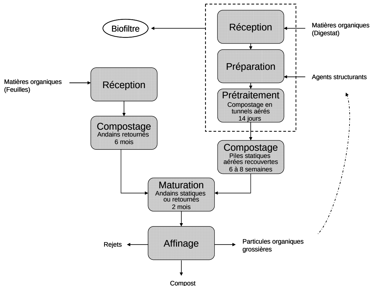
Figure 5.3 Schéma simplifié du concept de compostage en système semi-fermé
