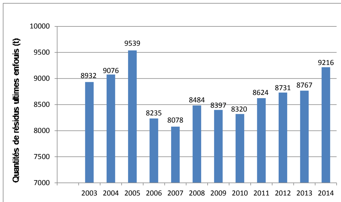
Figure 5 : Quantité de matières résiduelles éliminée via les collectes municipales de 2003 à 2014
