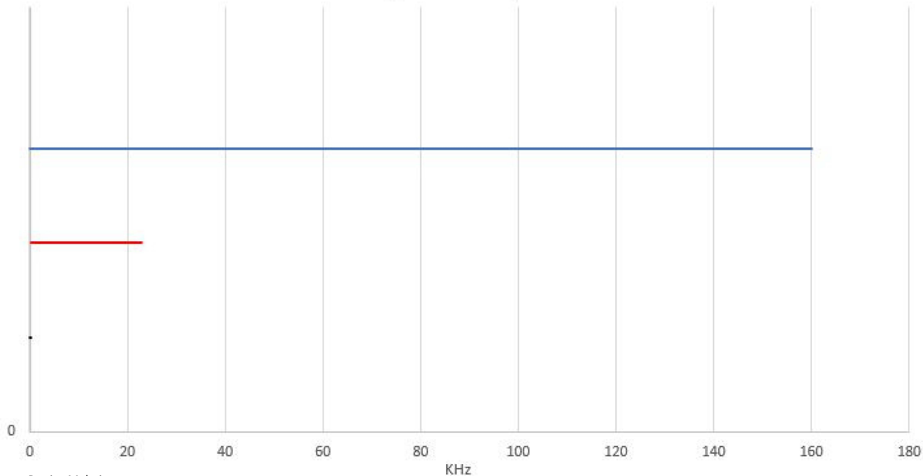
Figure 2 Plage audible du béluga versus plages de bruit des navires marchand et bateau à moteur hors bord (échelle linéaire)
