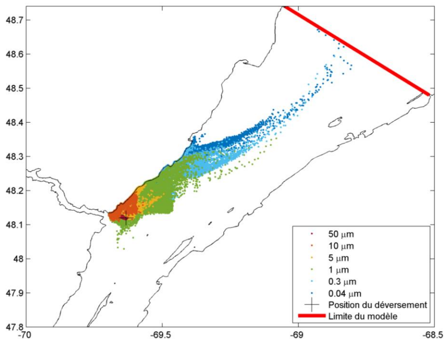
Figure 9 : Cumul des zones affectées par le déversement de diesel à l'embouchure du Saguenay en conditions de vent du sud-sud-ouest (après 120 heures) en fonction de l'épaisseur de la nappe d'hydrocarbure
