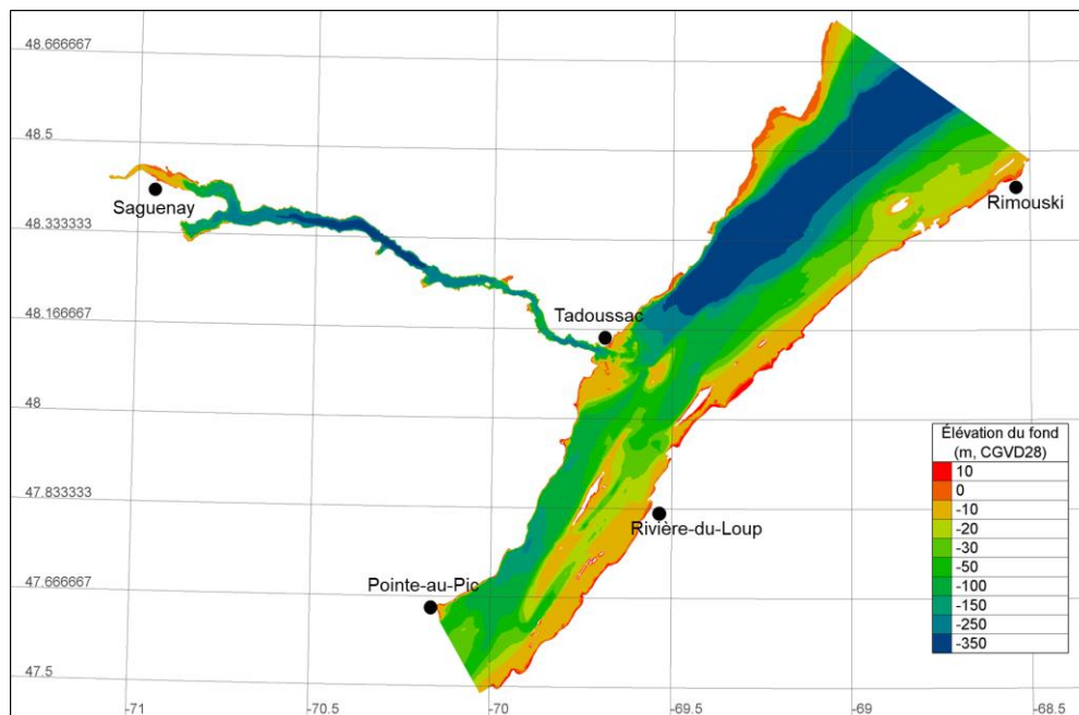
Figure 1 : Domaine de calcul pour le modèle hydrodynamique TELEMAC-3D
