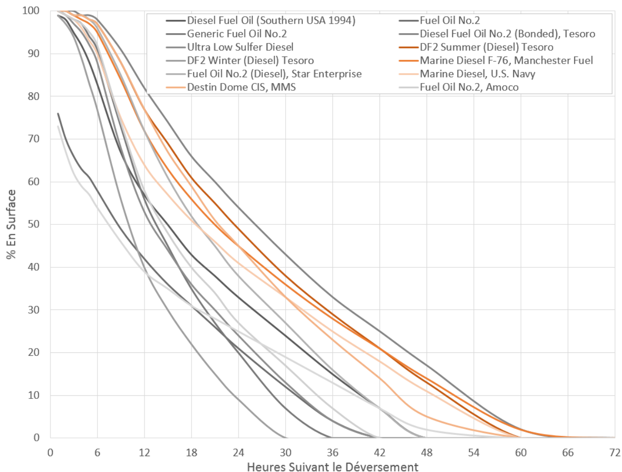
Figure 2 : Comportement sur l'eau de différents carburants de type MGO
