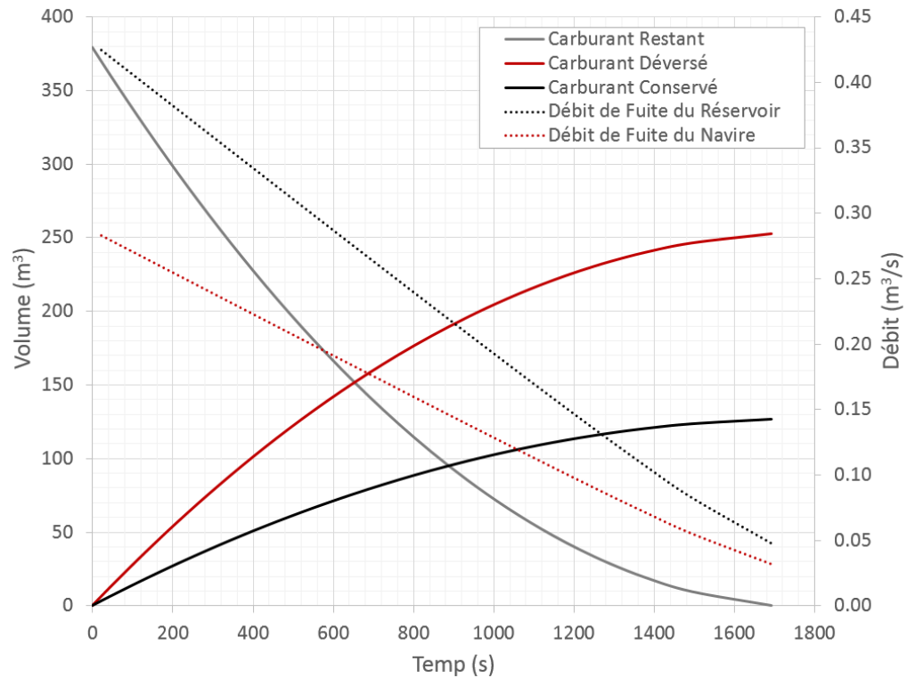
Figure 3 : Bilan de masse du déversement de carburant
