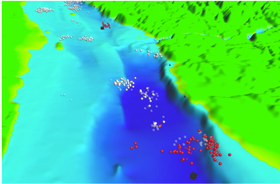
Figure 2: Capture d'écran d'une simulation de 3MTSim illustrant les interactions entre navires et bélugas dans l'estuaire du Saint-Laurent. Les cubes noirs sont des navires marchands et les sphères représentent des bélugas (rouges s'ils sont exposés à un niveau de bruit intégré (10-1122 Hz) supérieur à 120 dB re 1 \mu Pa, blancs sinon).
