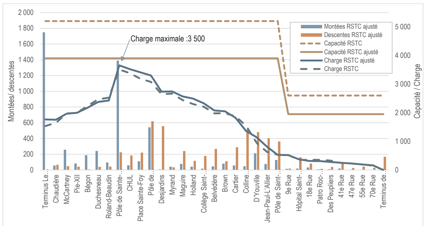
Figure 7 Profil de charge du tramway en direction est, à l'heure de pointe (7 h à 8 h), an 15
