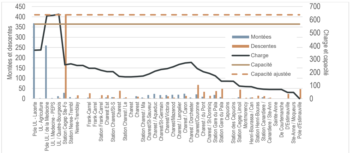
Figure 10 Profil de charge du Métrobus (axe du trambus Charest) en direction ouest avec le RSTC ajusté, à l'heure de pointe (7 h à 8 h), an 15
