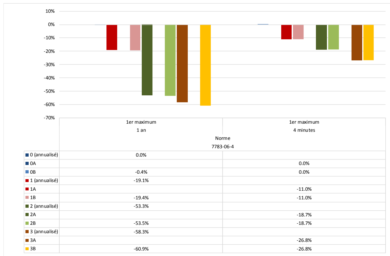
Figure 8 : Évolution des concentrations maximales de H 2 S modélisées par rapport au scénario de base
