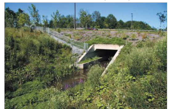
Figure 6-B : Passage à deux niveaux pour la petite faune.
