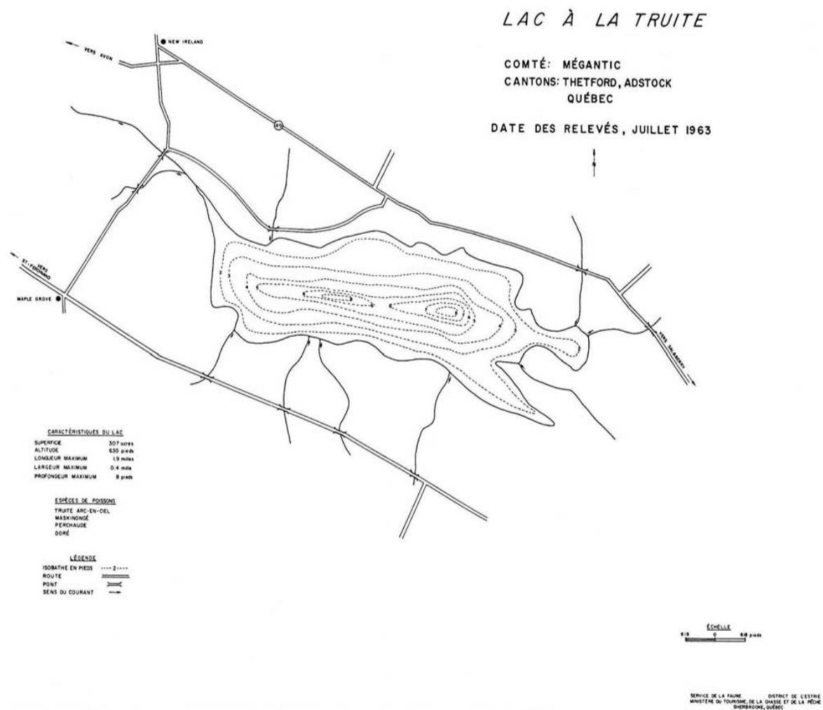
Carte 3 : Carte batymétrique du lac à la Truite d'Irlande, 1963
