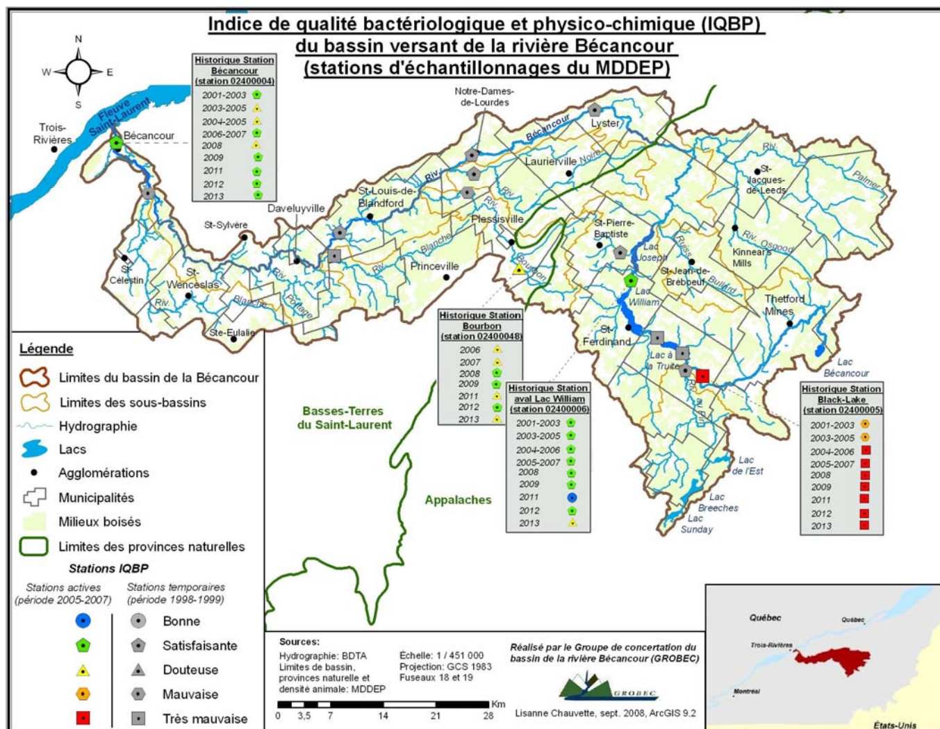
Carte 4 : Indice de qualité bactériologique et physico-chimique (IQBP) du bassin versant de la rivière Bécancour (GROBEC, comm. personnelle)
