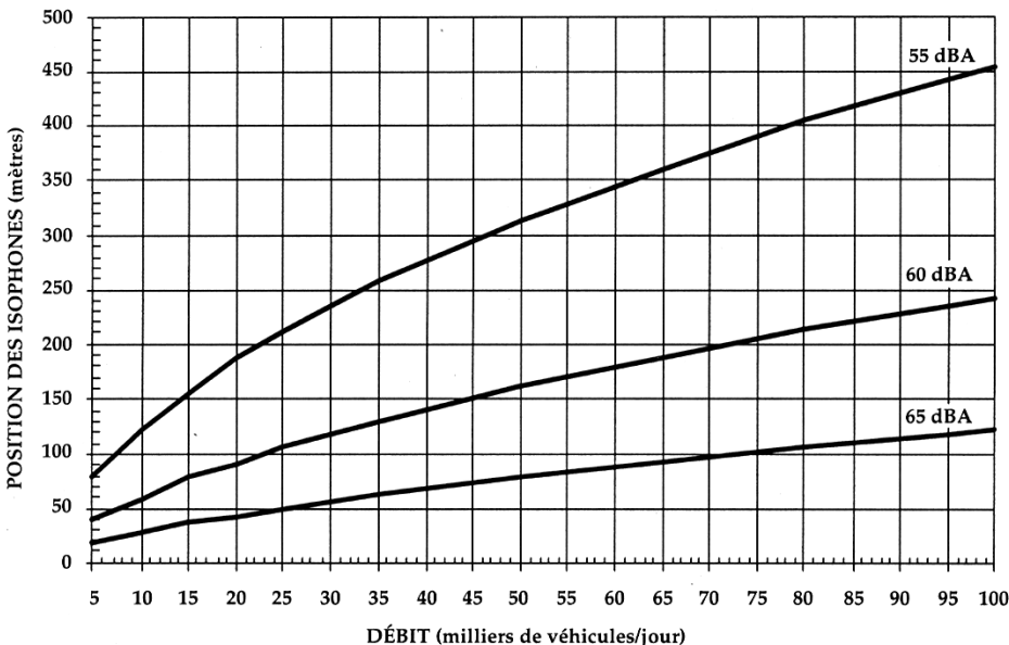
Illustration DC8-2 – Isophones projetées pour une vitesse de 90 km/h
