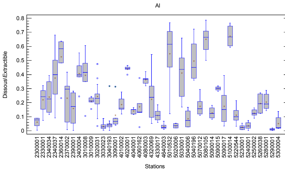
(b) Distribution des ratios dissous/extractible pour l'aluminium aux 41 stations
