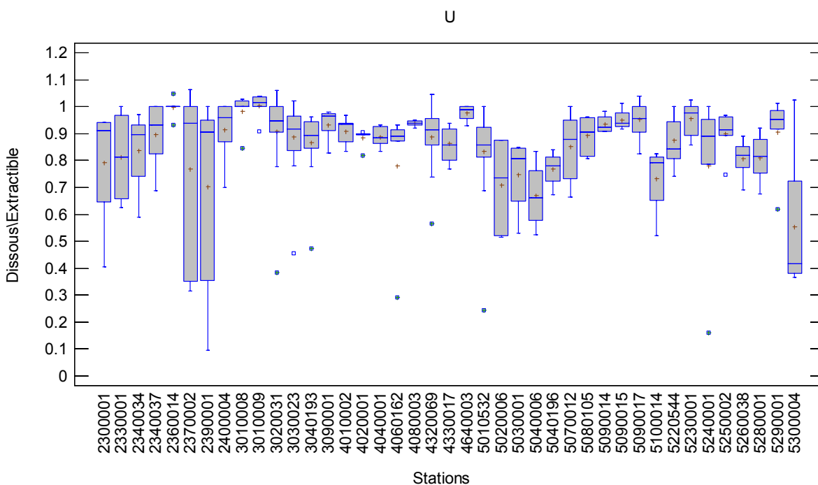
(r) Distribution des ratios dissous/extractible pour l'uranium aux 41 stations
