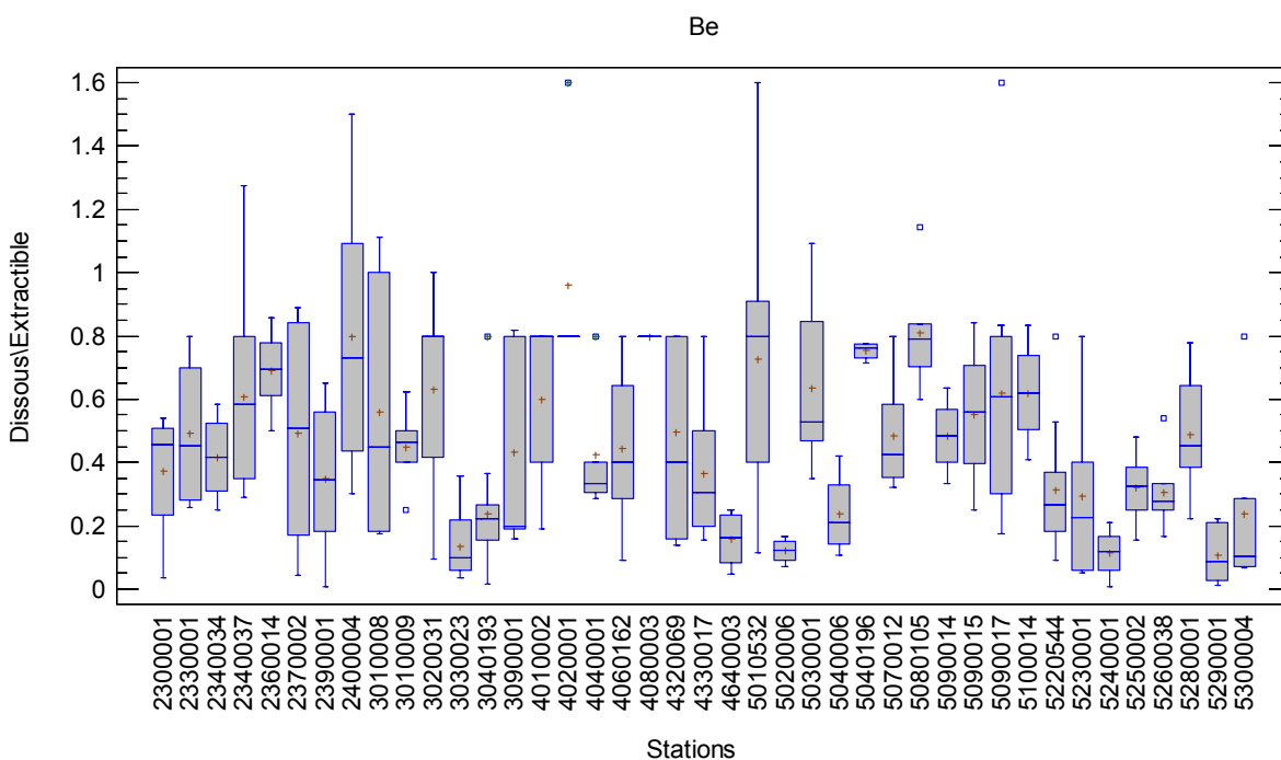
(f) Distribution des ratios dissous/extractible pour le béryllium aux 41 stations
