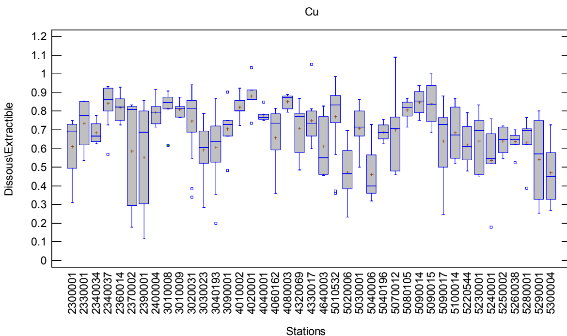
(j) Distribution des ratios dissous/extractible pour le cuivre aux 41 stations
