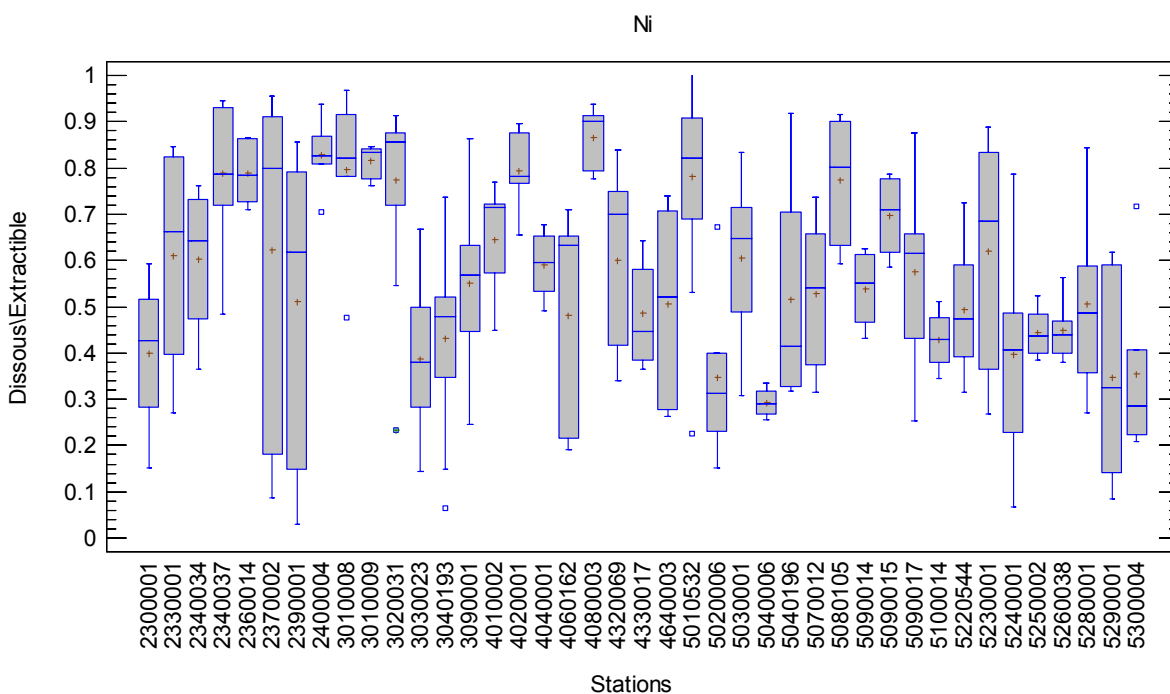
(n) Distribution des ratios dissous/extractible pour le nickel aux 41 stations
