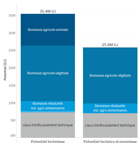
Figure 4 : Potentiels technique et technico-économique en 2018
