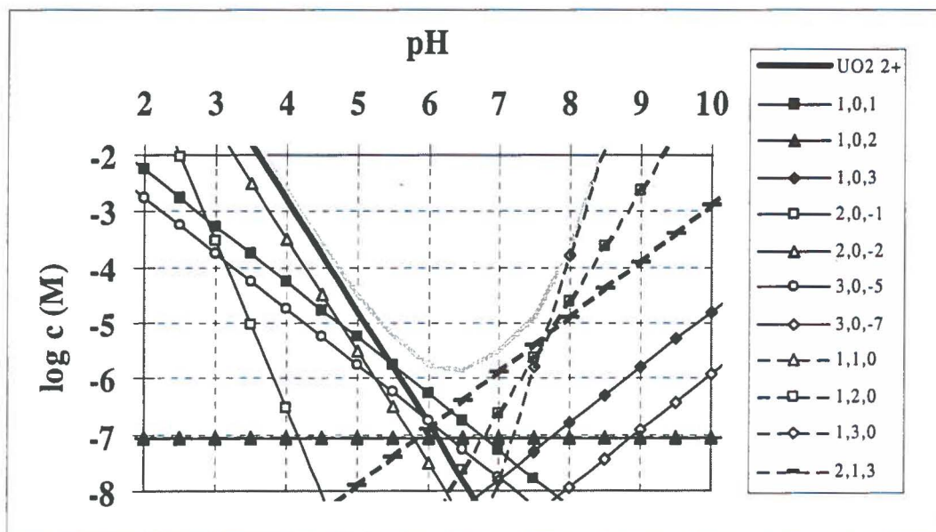
Figure 2 Spéciation de l'U(+6) en fonction du pH en équilibre avec le \text{CO}_2 de l'air et de la calcite avec une force ionique de 0.375 M. La ligne grise indique la concentration maximale d'U(+6) dissout (pourvu qu'il y a assez de l'U(+6) à disponible, BD1, x,y,z : x = U(+6), y = carbonate, z = hydroxyle).
