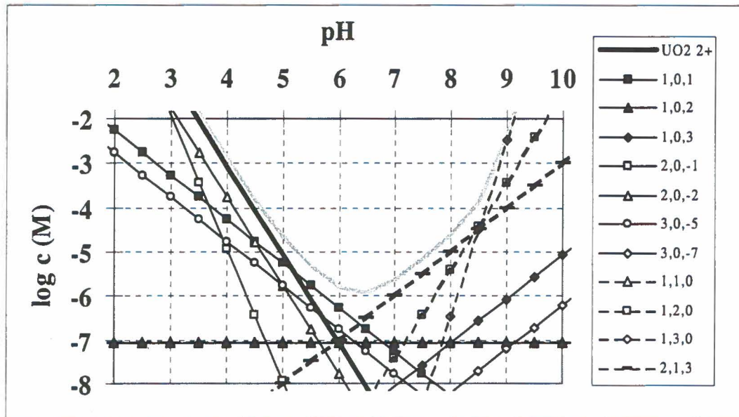
Figure 1 Spéciation de l'uranyle en fonction du pH en équilibre avec le \text{CO}_2 de l'air et de la calcite avec une force ionique de zéro. La ligne grise indique la concentration maximale d'U(+6) dissout (pourvu qu'il y a assez de l'U(+6) à disponible, BD1, x,y,z : x = U(+6), y = carbonate, z = hydroxyle).
