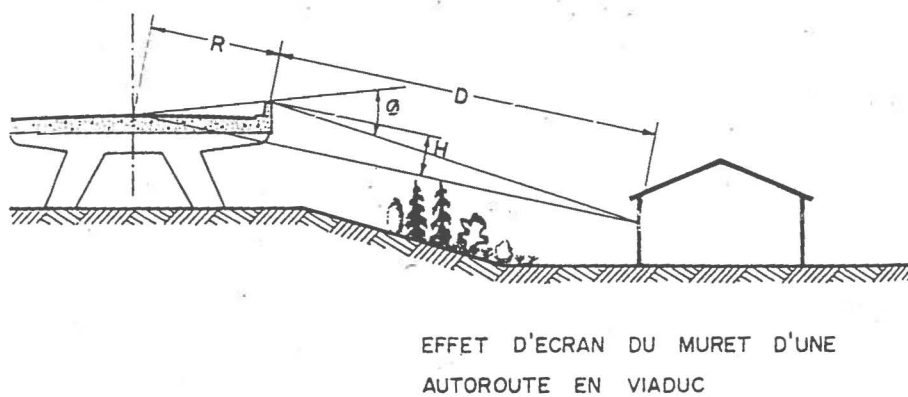
FIGURE No 78 Différents exemples d'effet d'écran au voisinage d'une autoroute — Paramètres de calcul.
