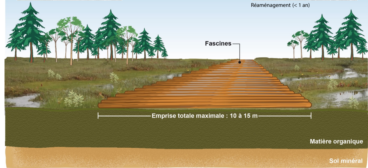
Figure A.3 : Sentier sur fascines
