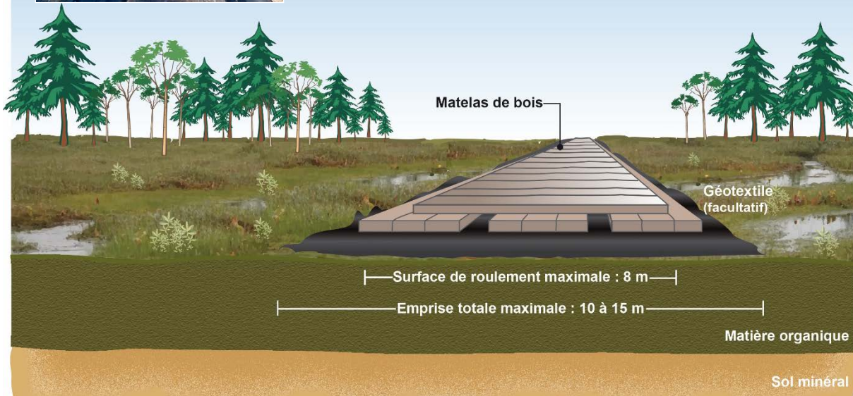
Figure A.8 : Chemin sur matelas de bois avec ou sans membrane géotextile
