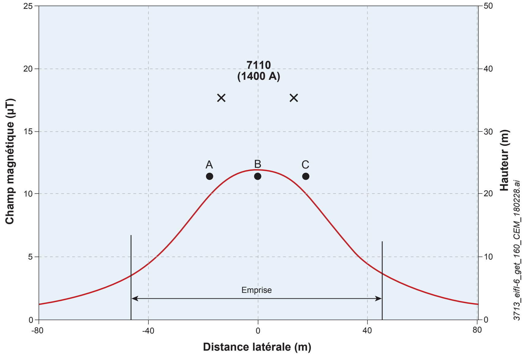
Figure I-6 Profil de CM sous la ligne 7110 (situation future)
